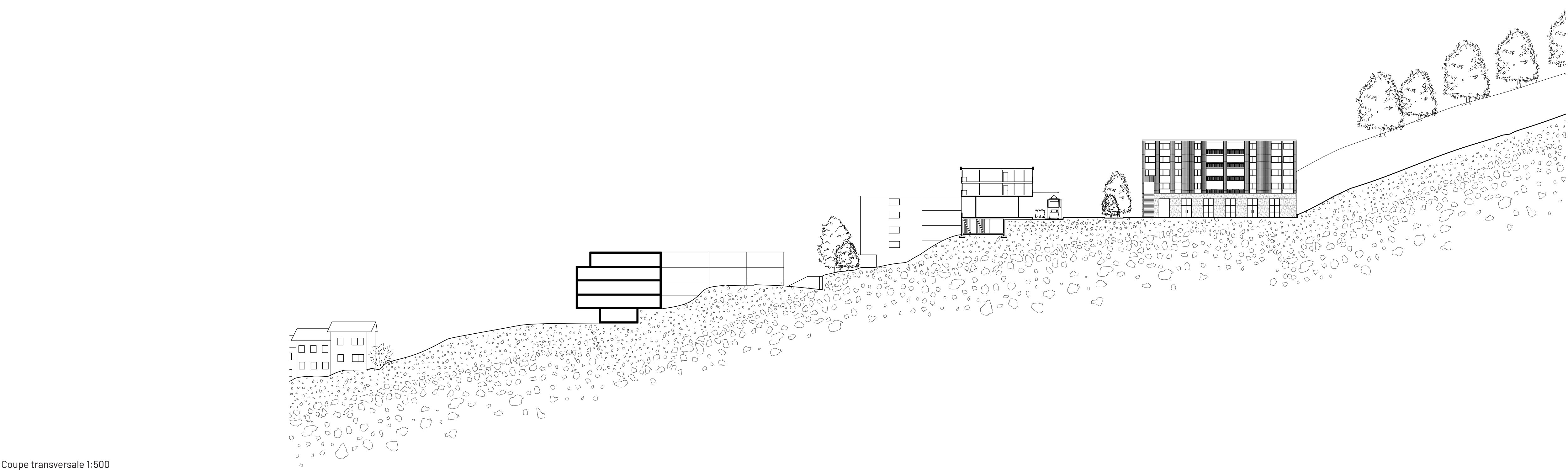
Coupe transversale 1:500
