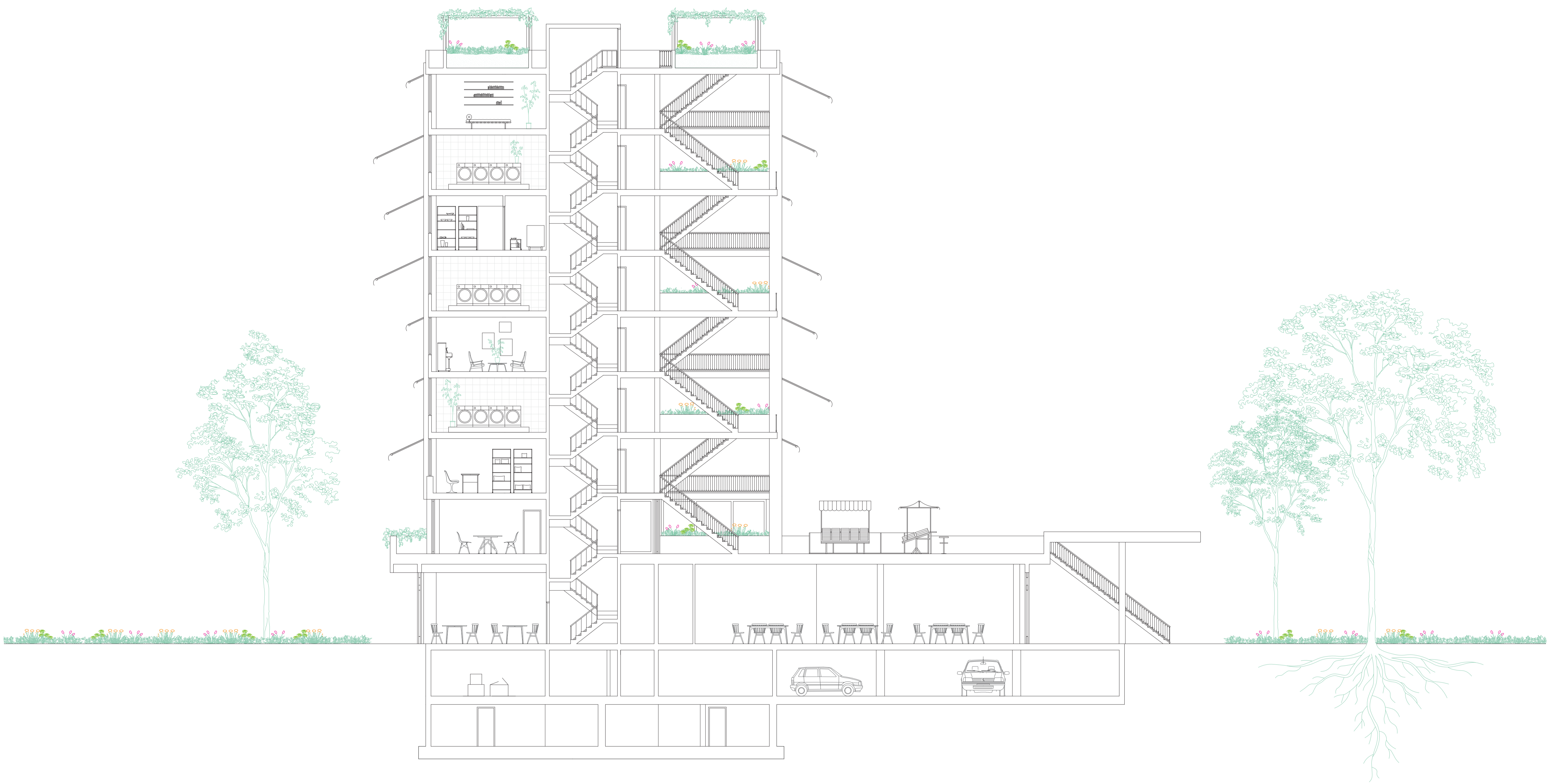
Coupe transversale
