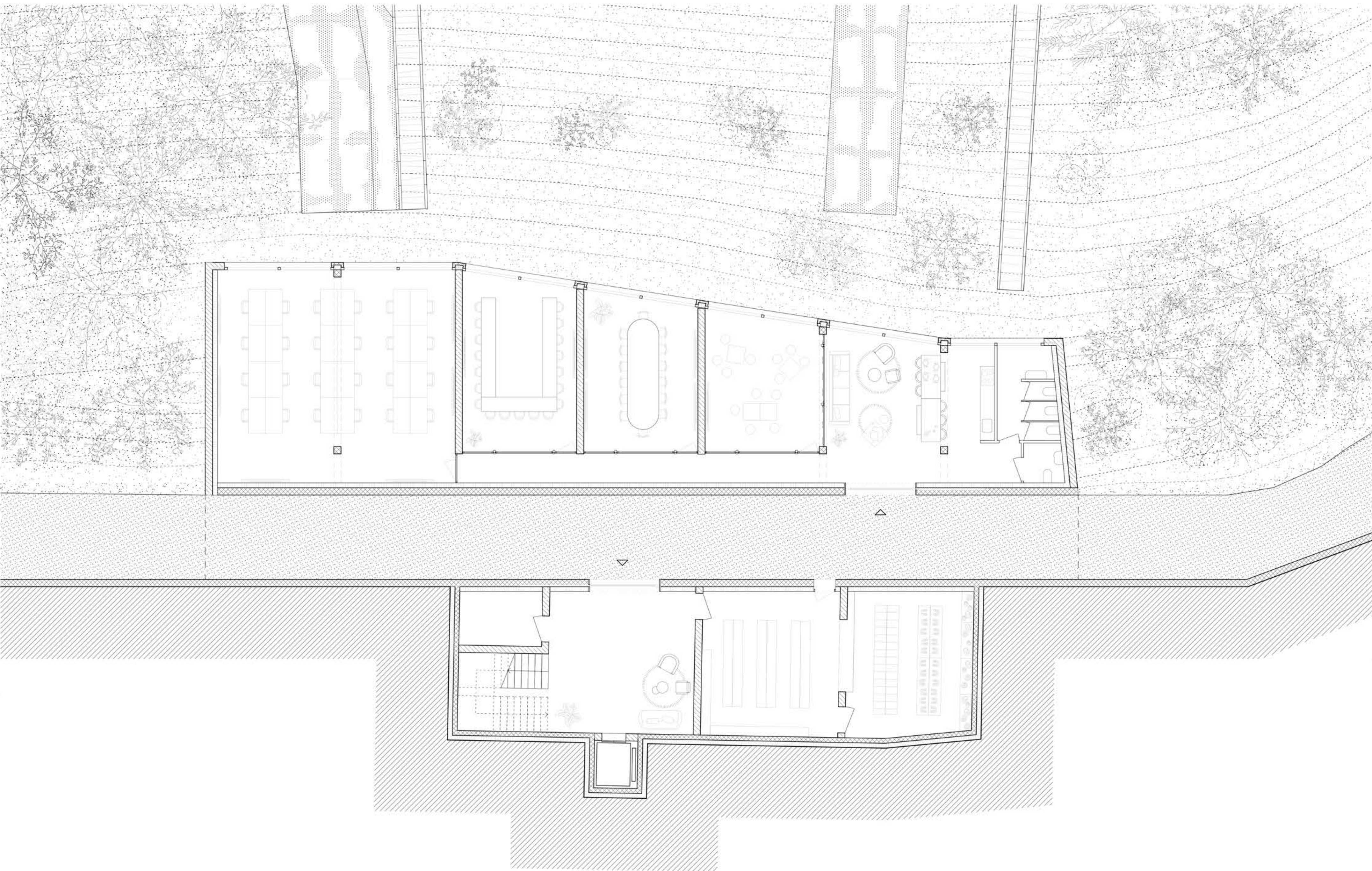
Plan Rez-de-chaussée 1:100
