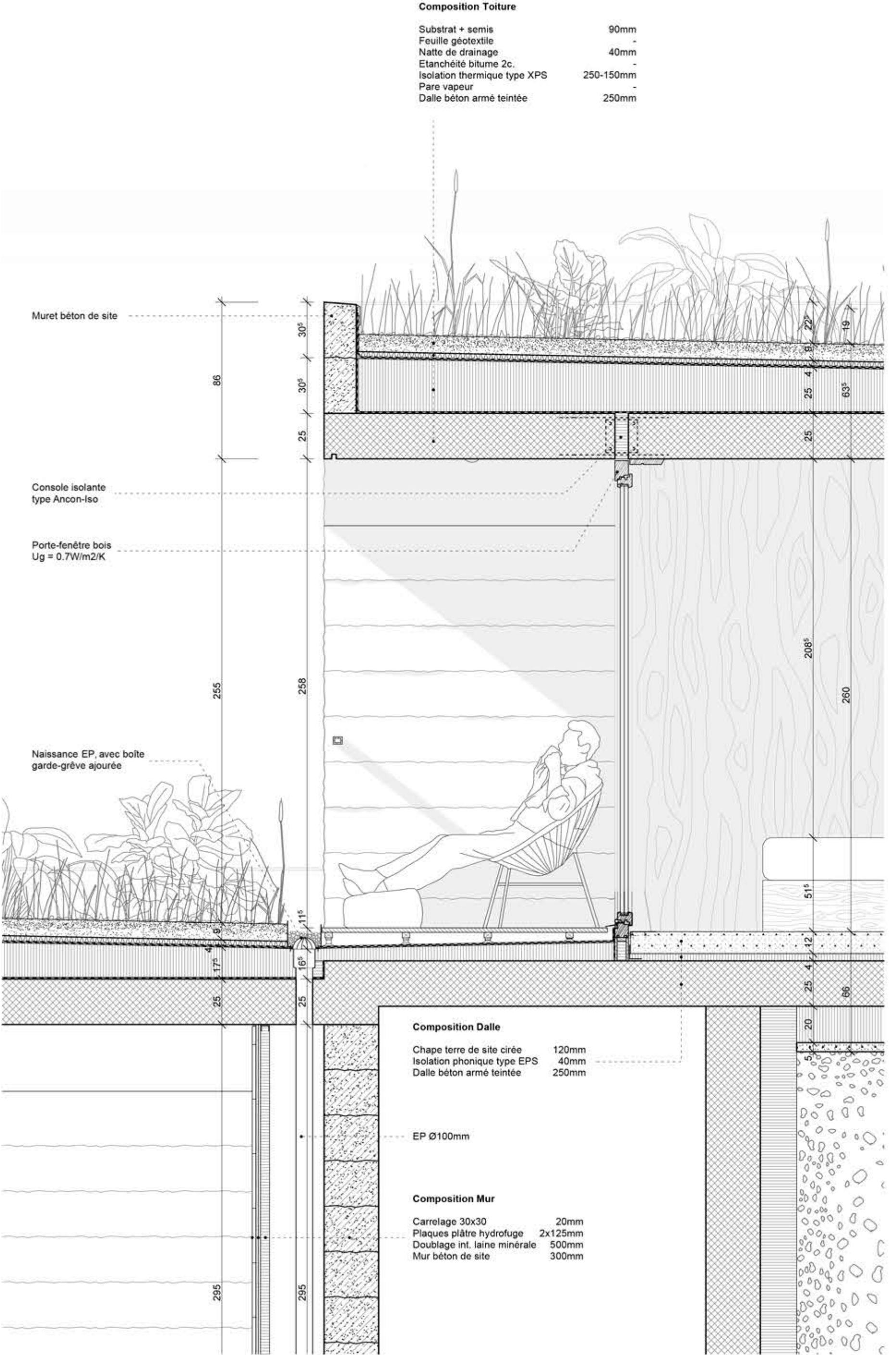
Coupe 1:20
