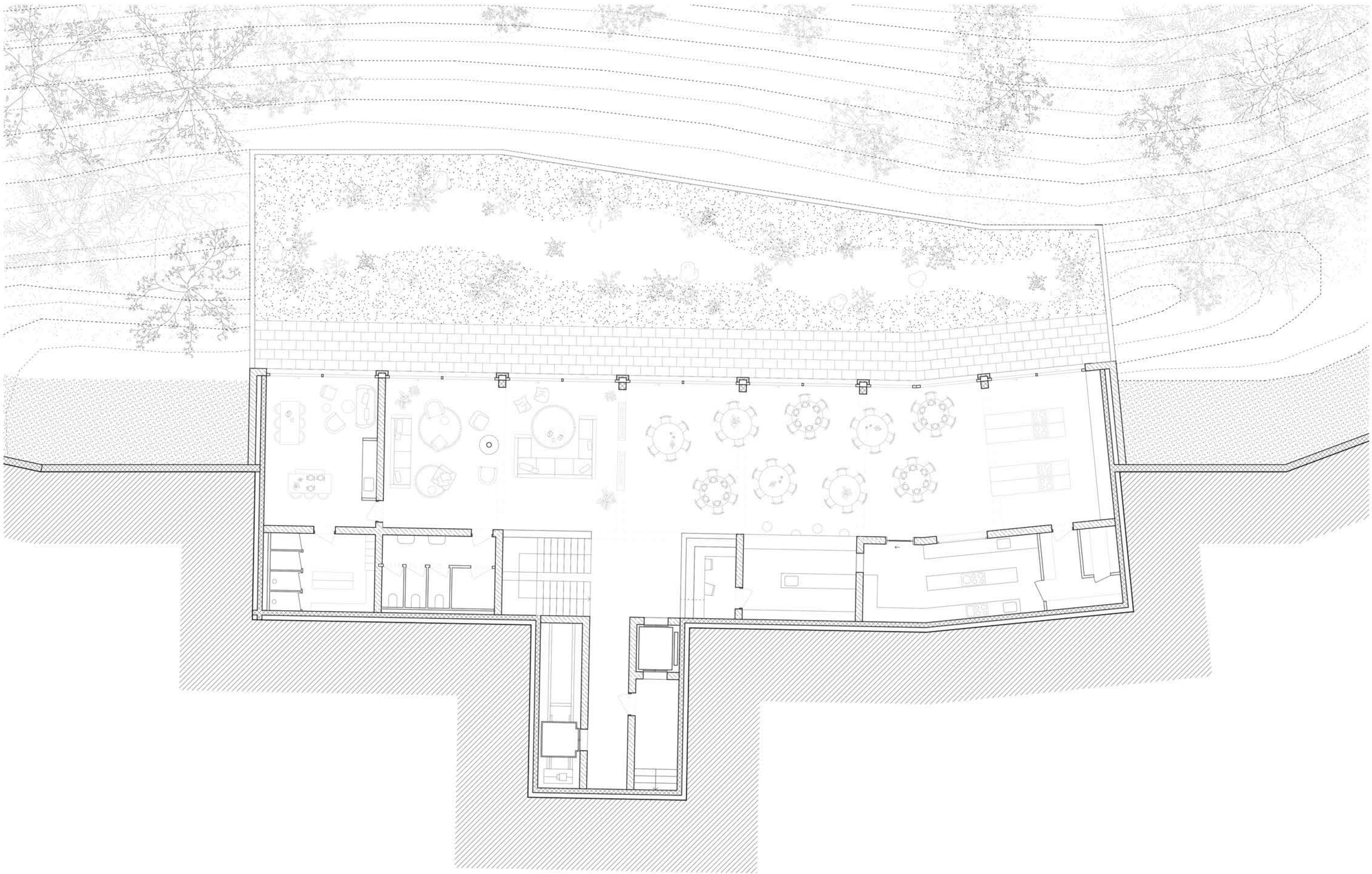
Plan premier étage 1:100
