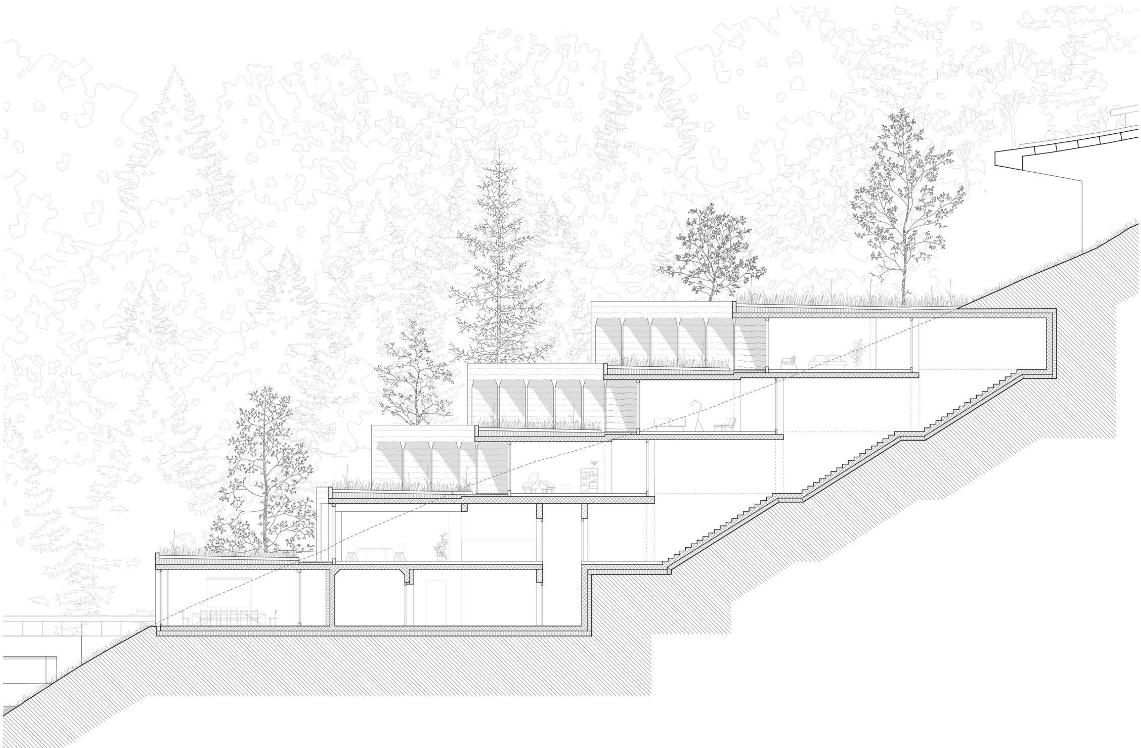
Coupe latérale 1:100
