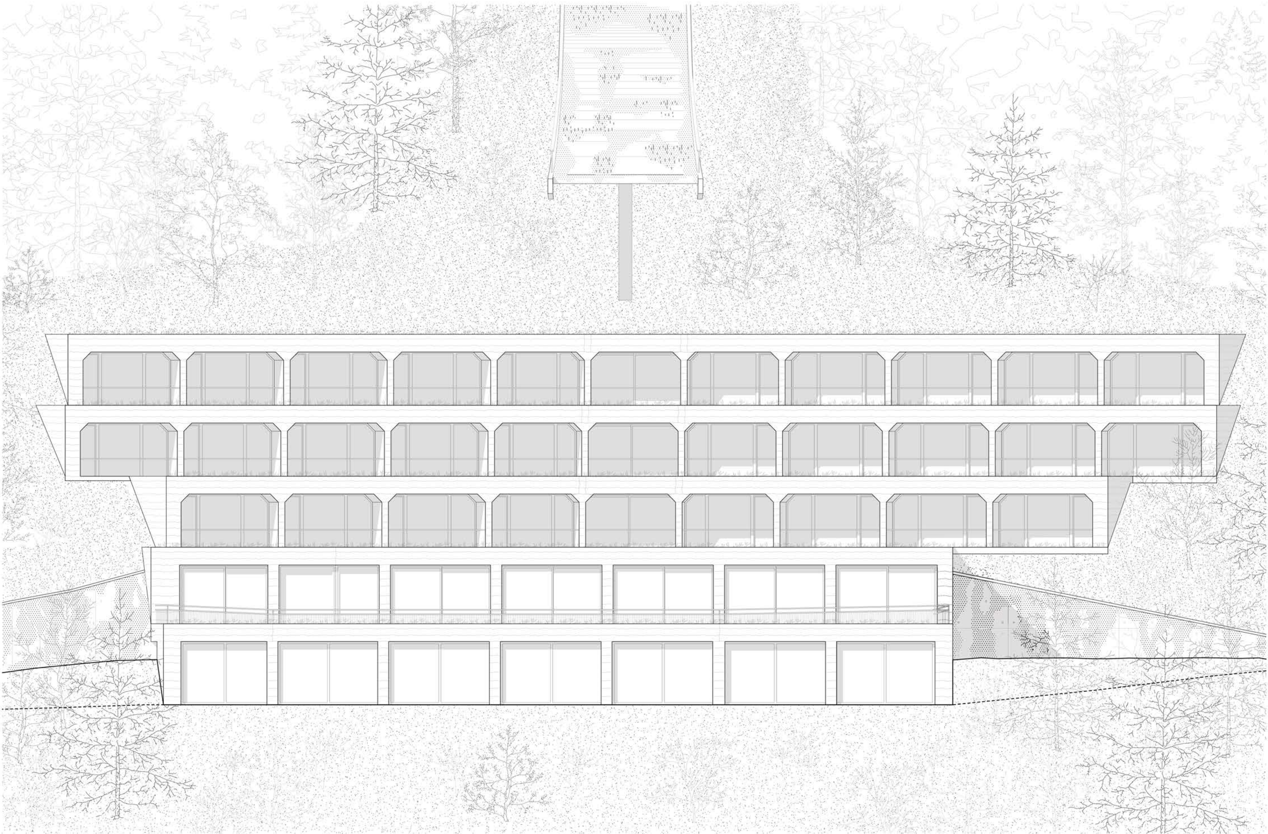
Elévation Nord-Est 1:100
