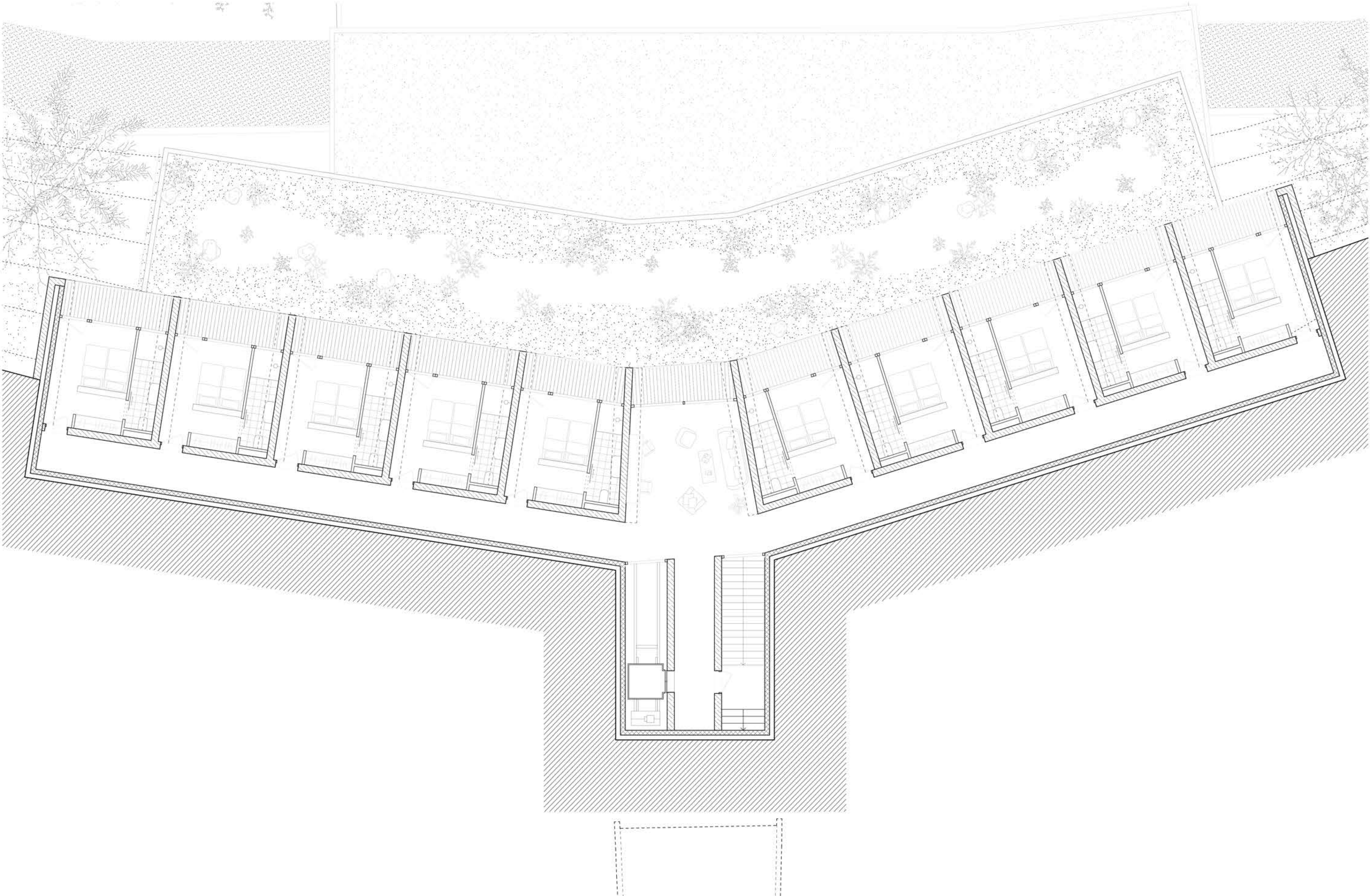
Plan troisième étage 1:100
