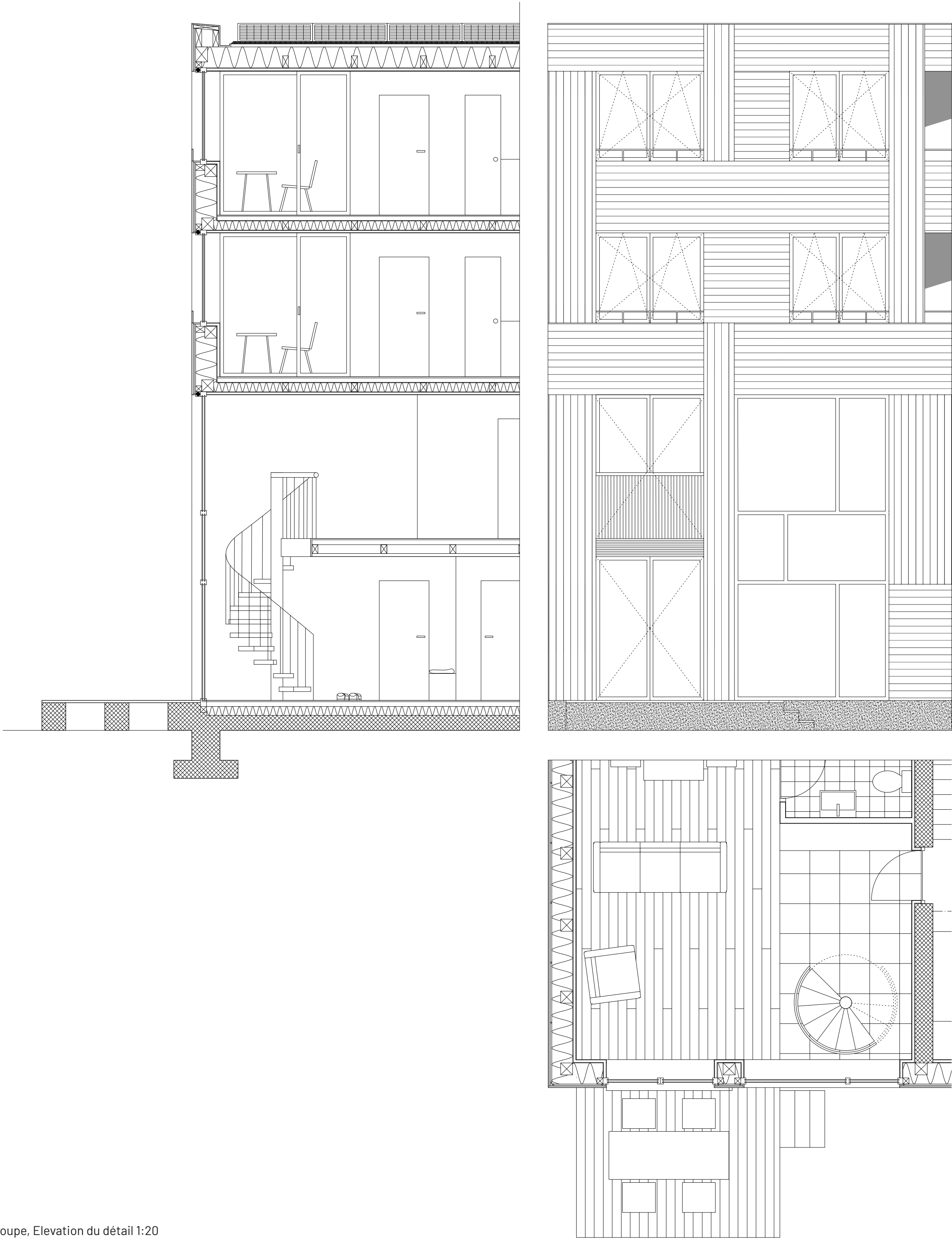
Plan, Coupe, Elevation du détail 1:20
