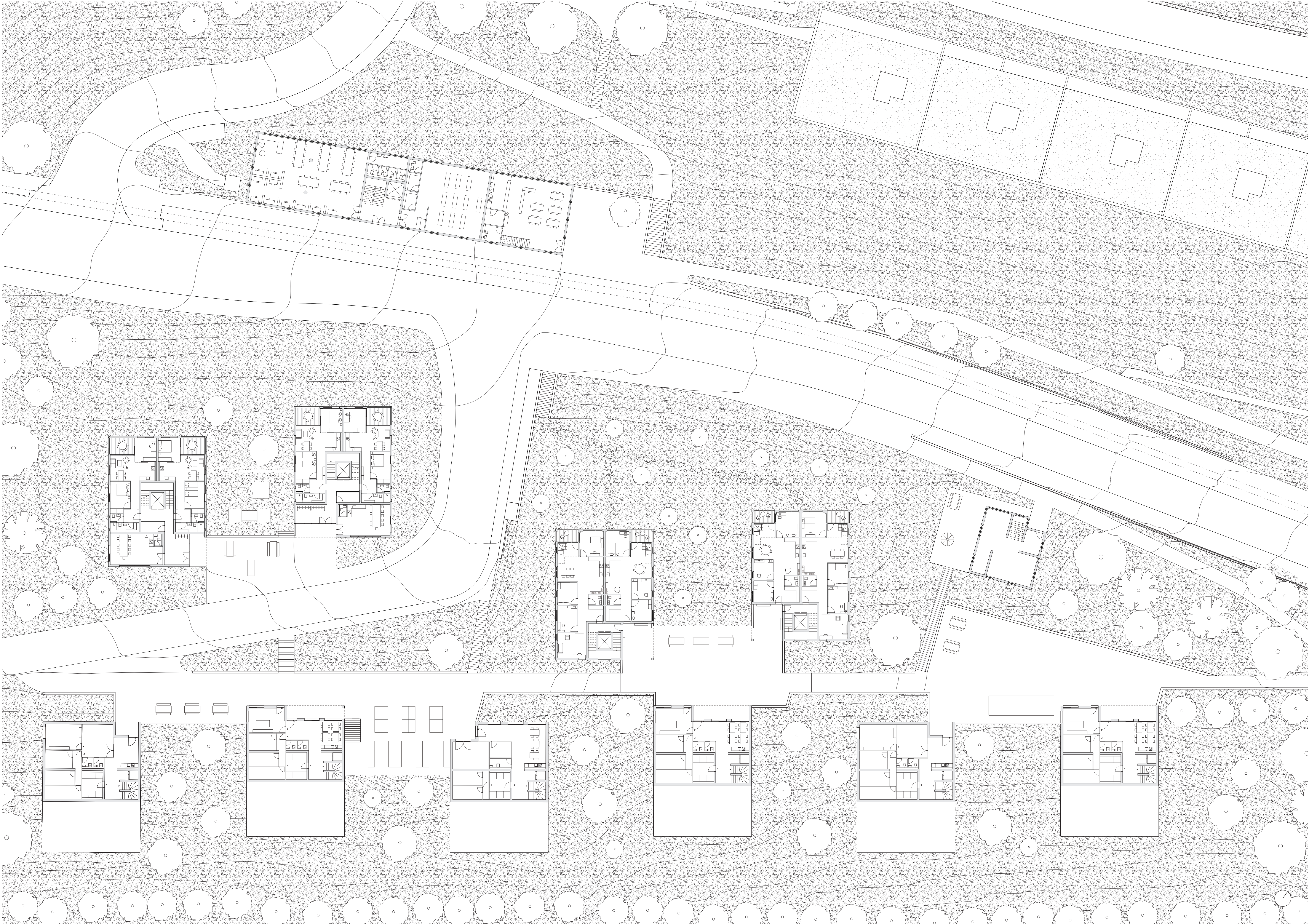
Plan des rez 1:250
