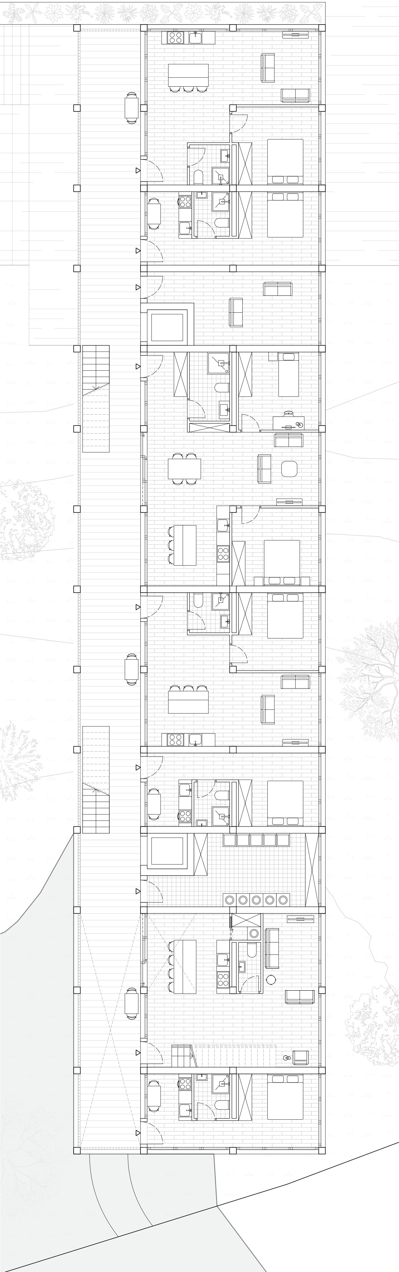
Niveau +3
