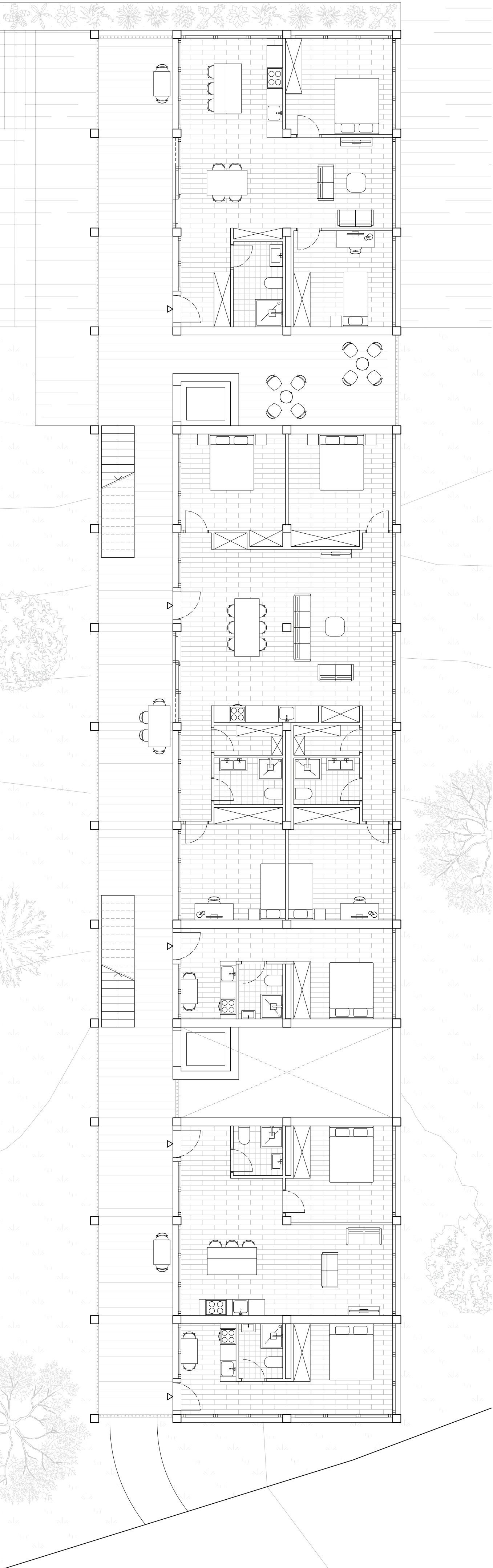
Niveau +5
