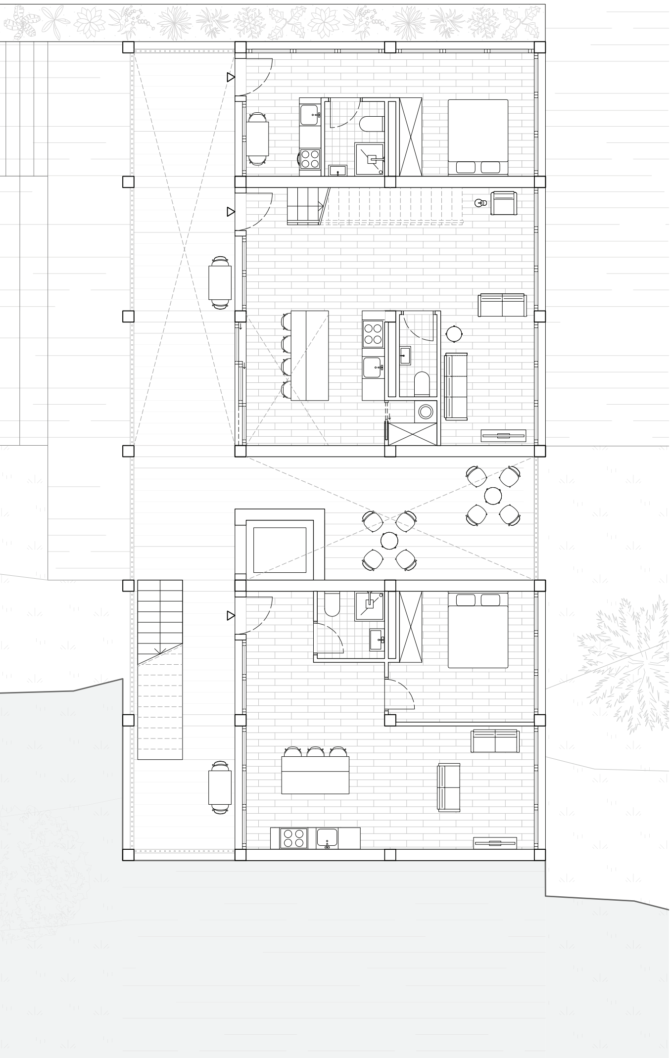
Niveau +1
