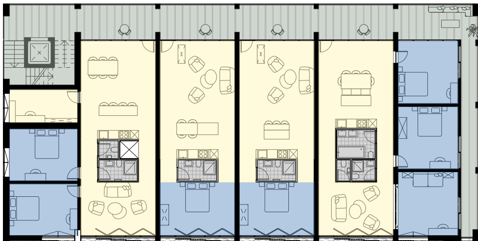
Schéma des zones d'un étage type
