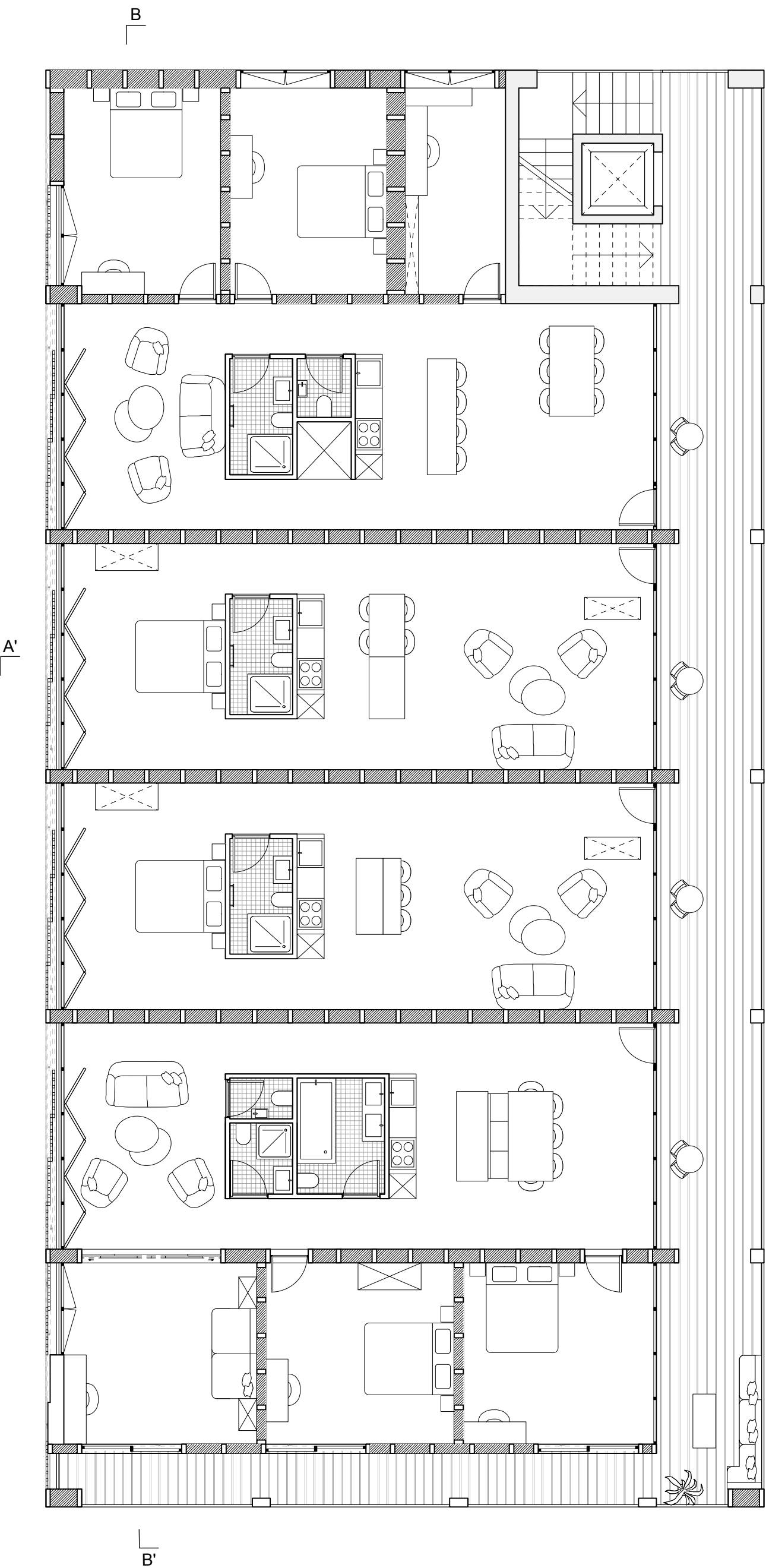
Plan 1:100 d'un étage type
