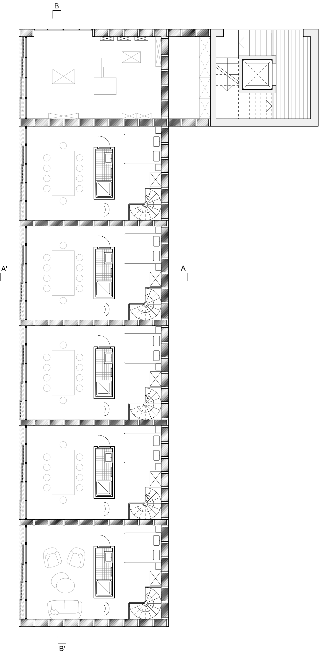
Plan 1:100 du premier étage
