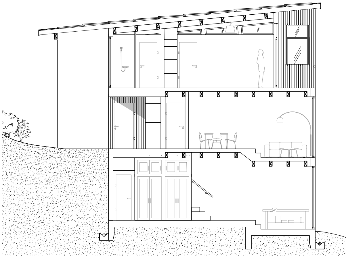
Coupe transversale Triplex, échelle 1:100
