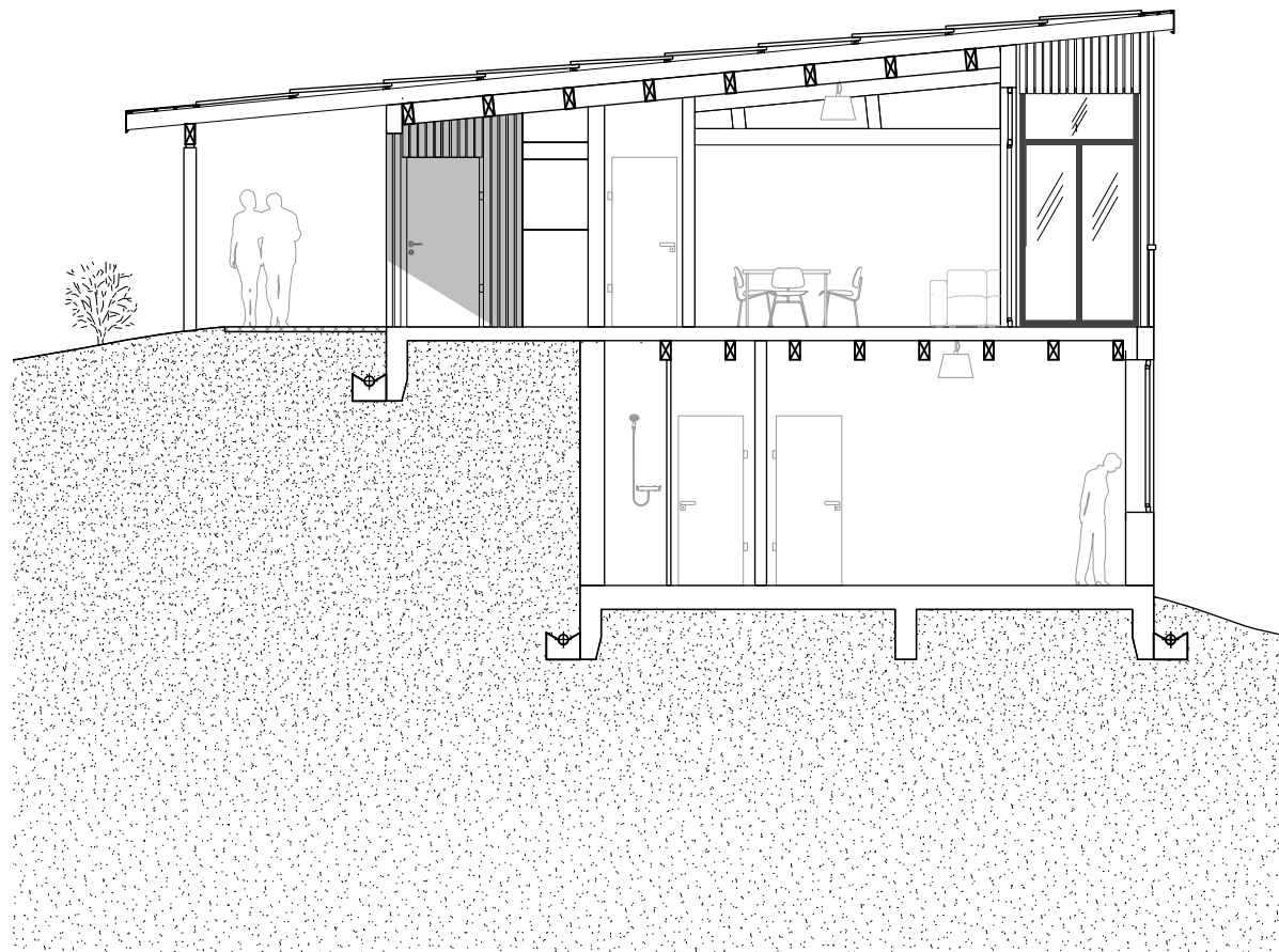
Coupe transversale Duplex, échelle 1:100
