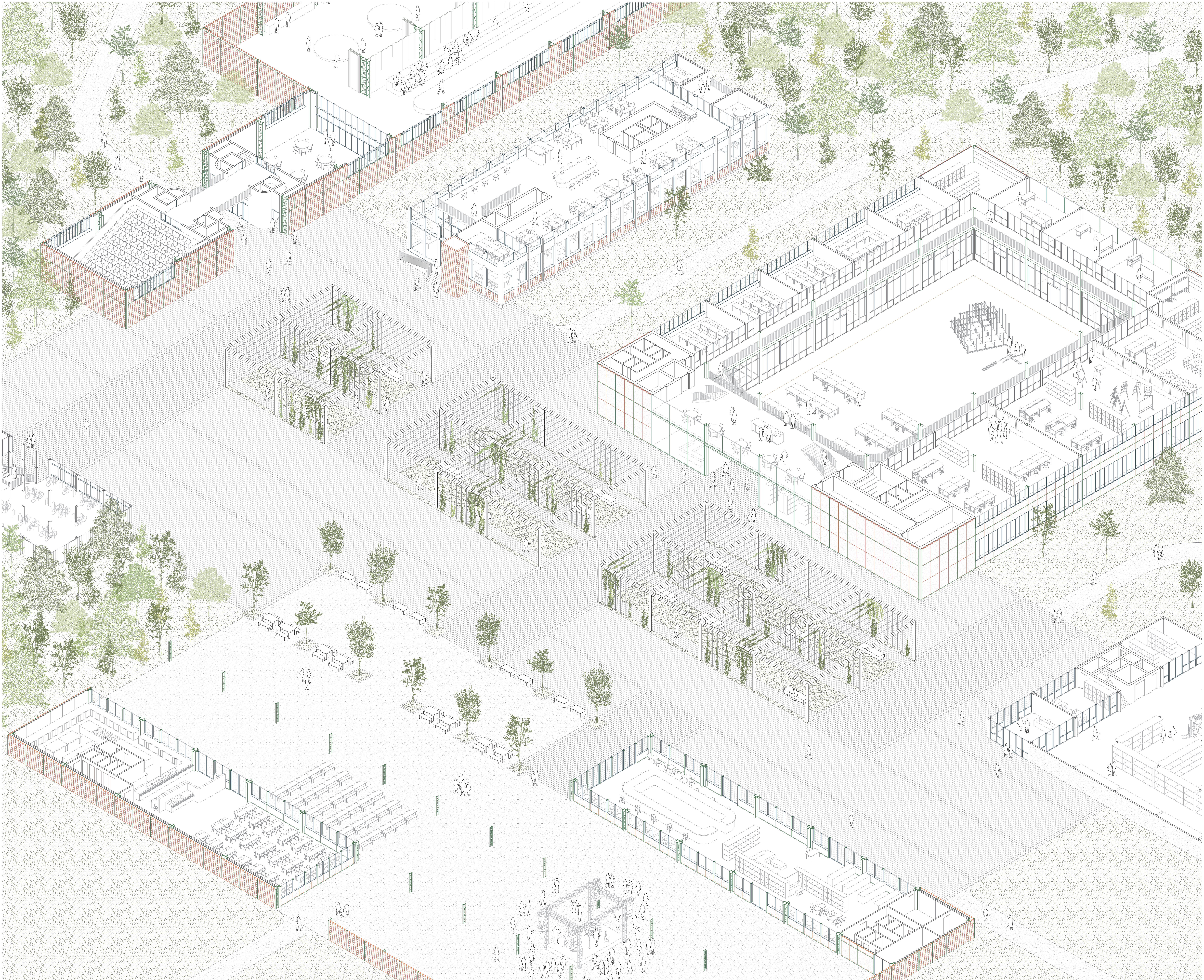
Axonométrie Interface entre les espaces collectifs extérieurs et intérieurs
