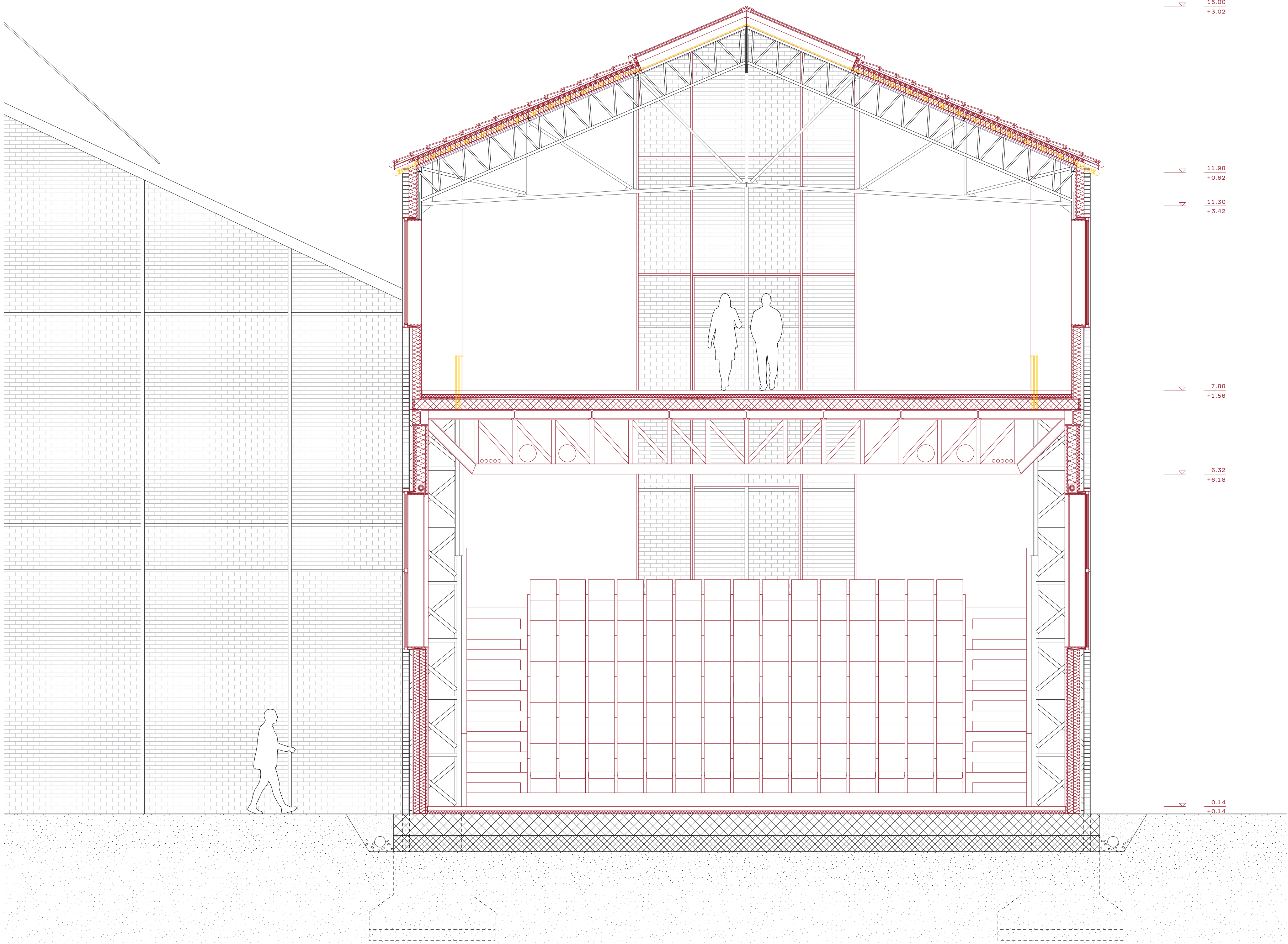
Coupe halle ouest (CC') Espaces de représentations artistiques — 1:50
