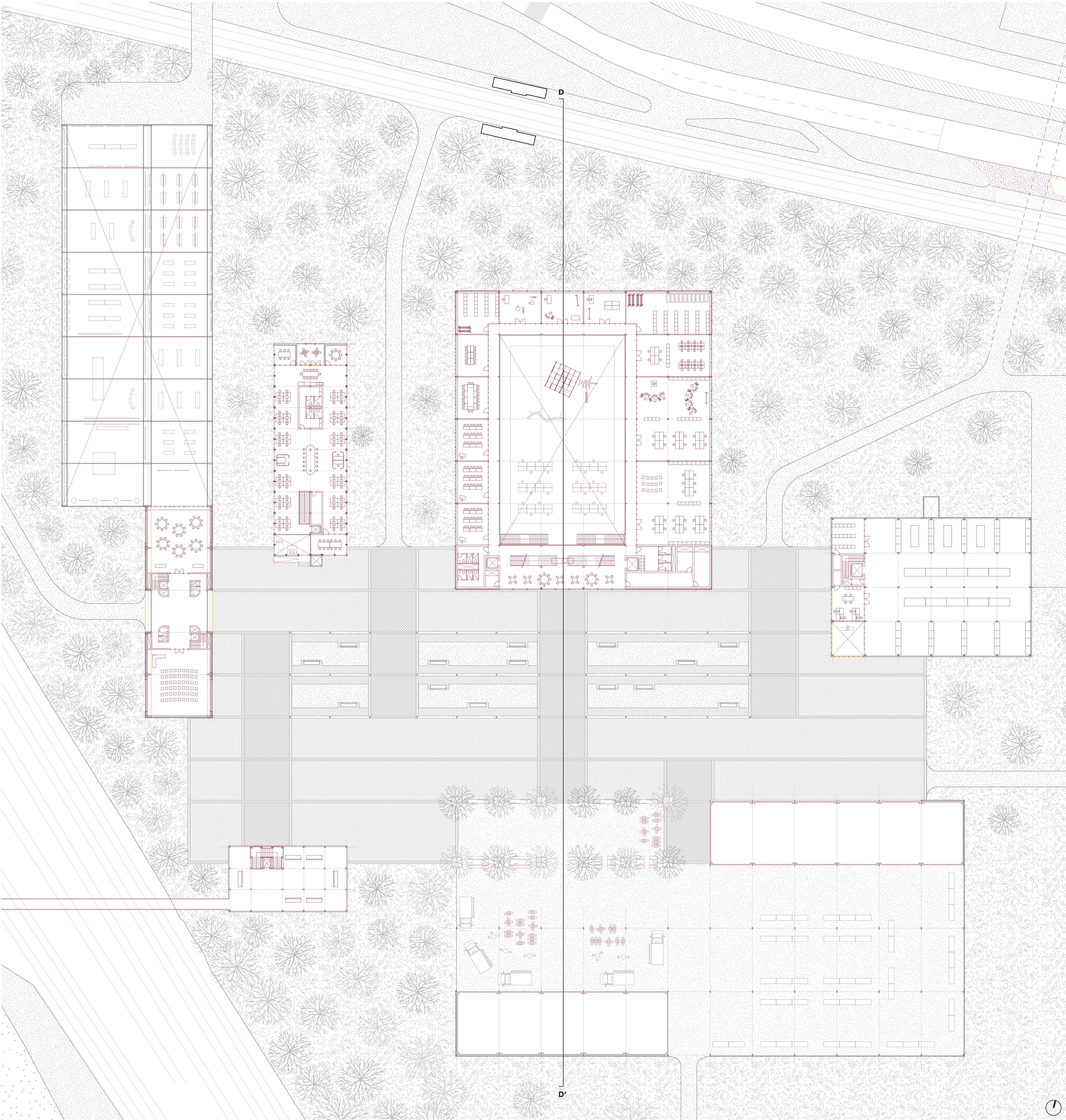
Plan 1 er étage — 1:300
