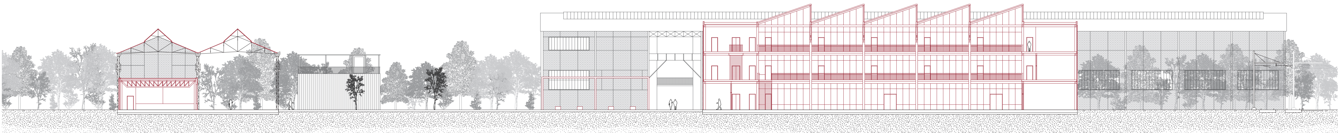
Coupe nord - sud (DD') Relation entre la place et les bâtiments du site — 1:300
