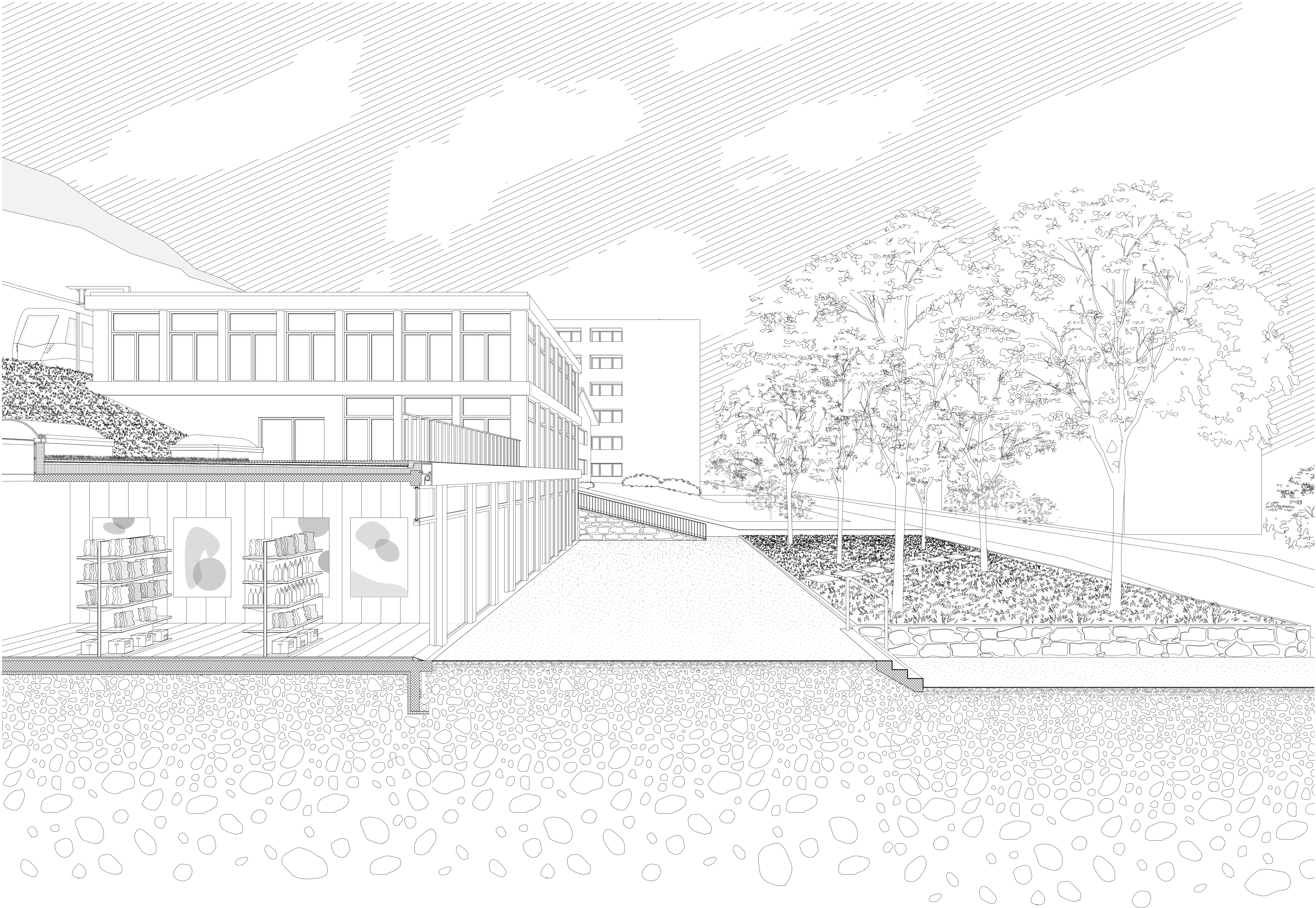
Coupe perspective de la place de la gare 1:30
