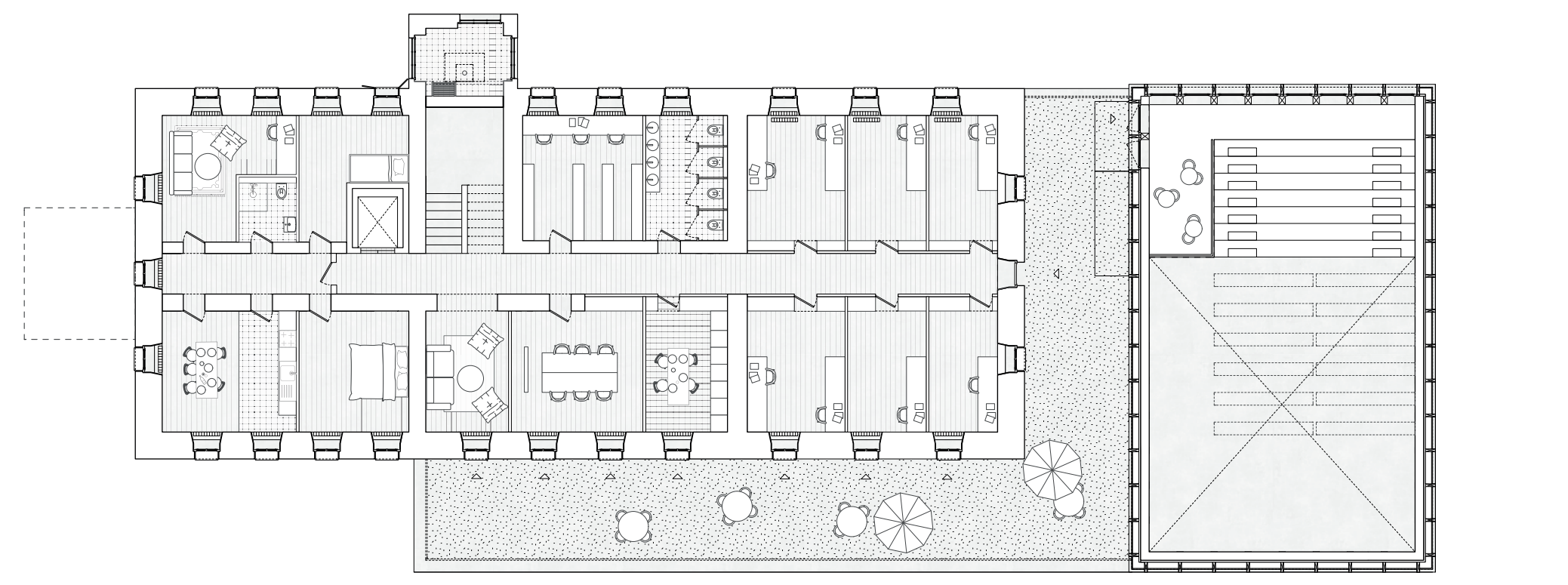
Plan 1er étage
