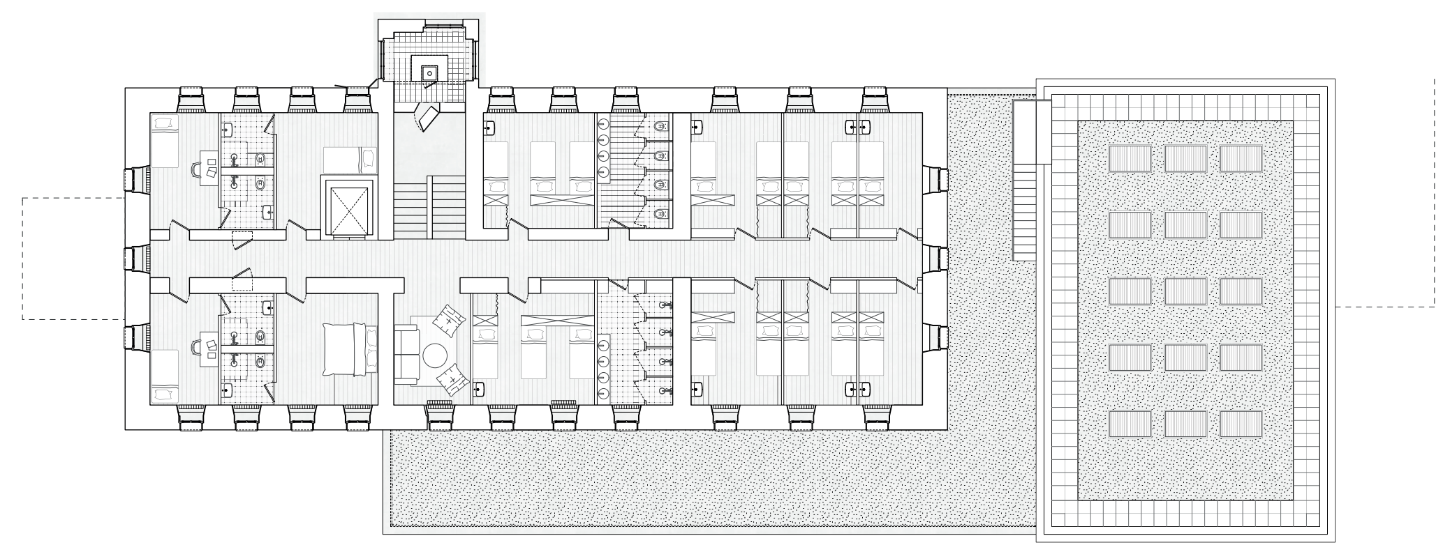
Plan 2ème, 3ème et 4ème étage
