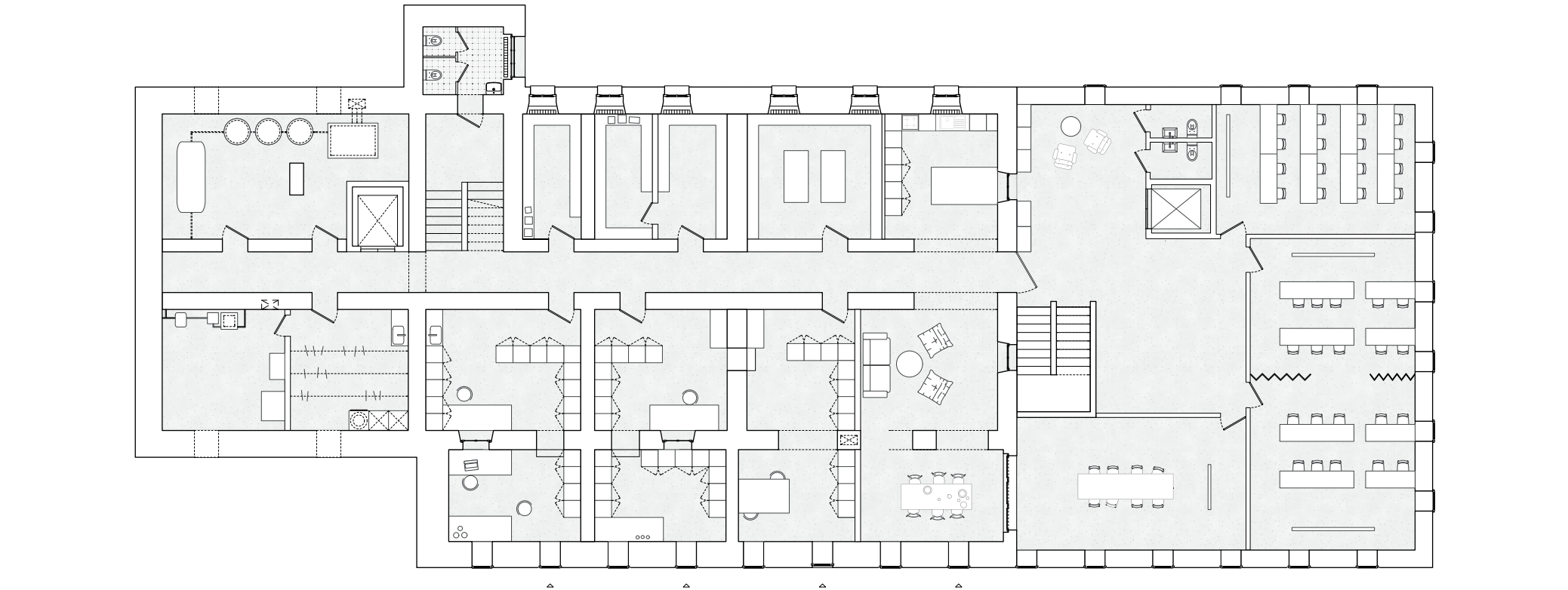
Plan rez de chaussée inférieur
