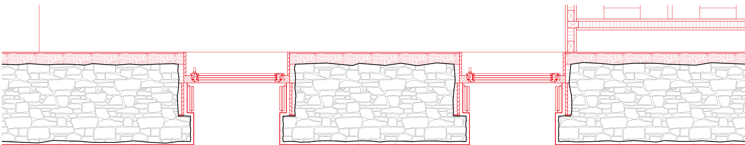
Détail façade Nord-Est - 1:20
