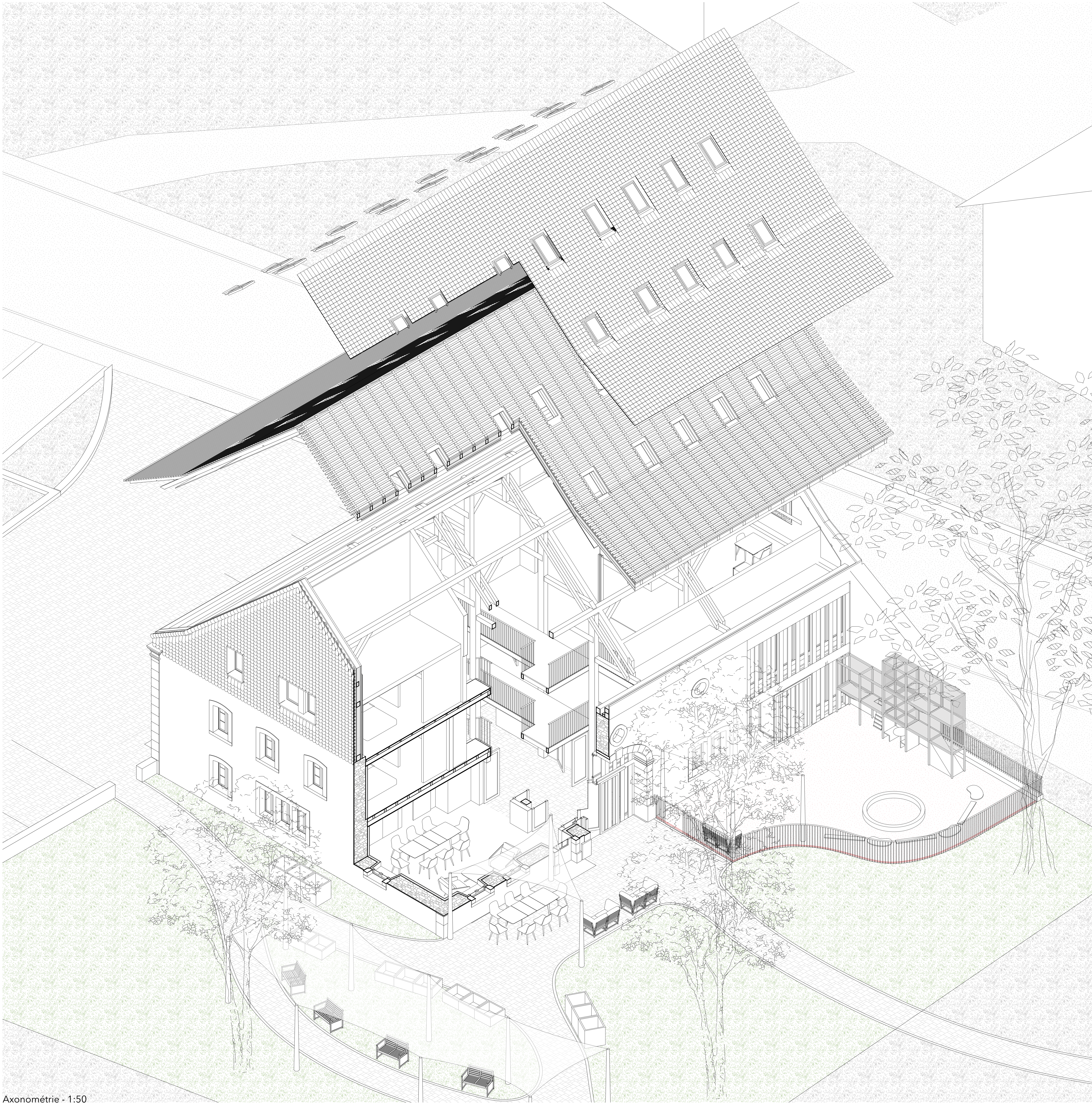
Axonométrie - 1:50
