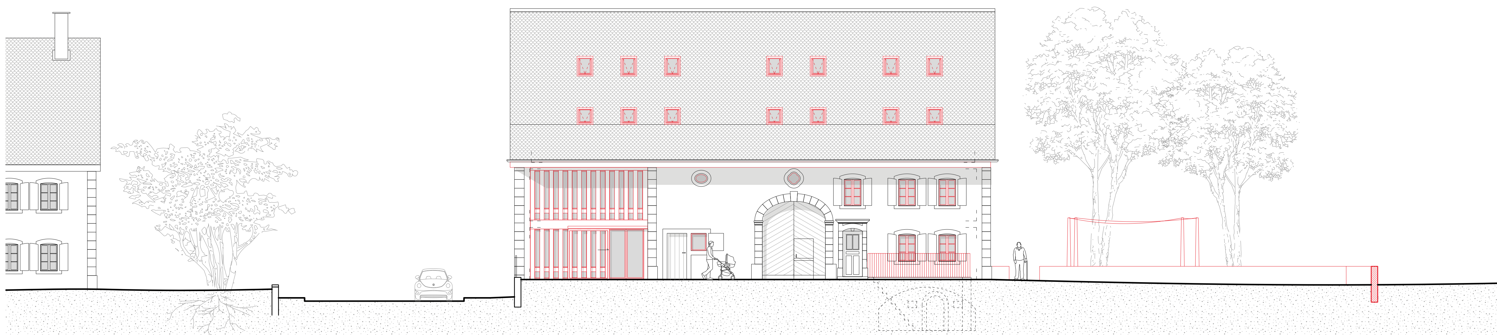
Façade Nord-Ouest - 1:100
