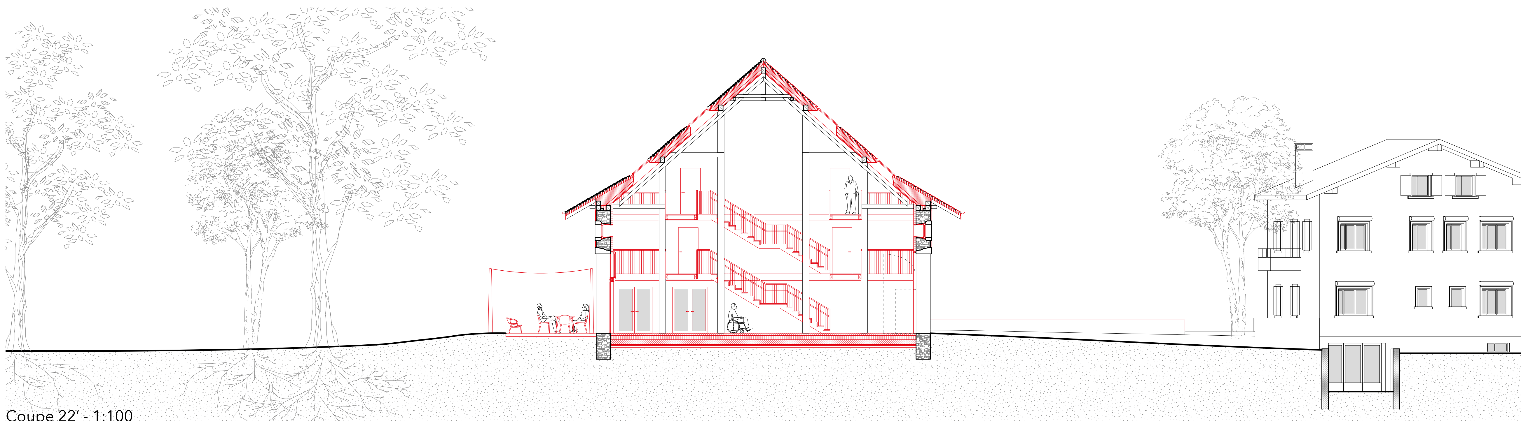
Coupe 22' - 1:100
