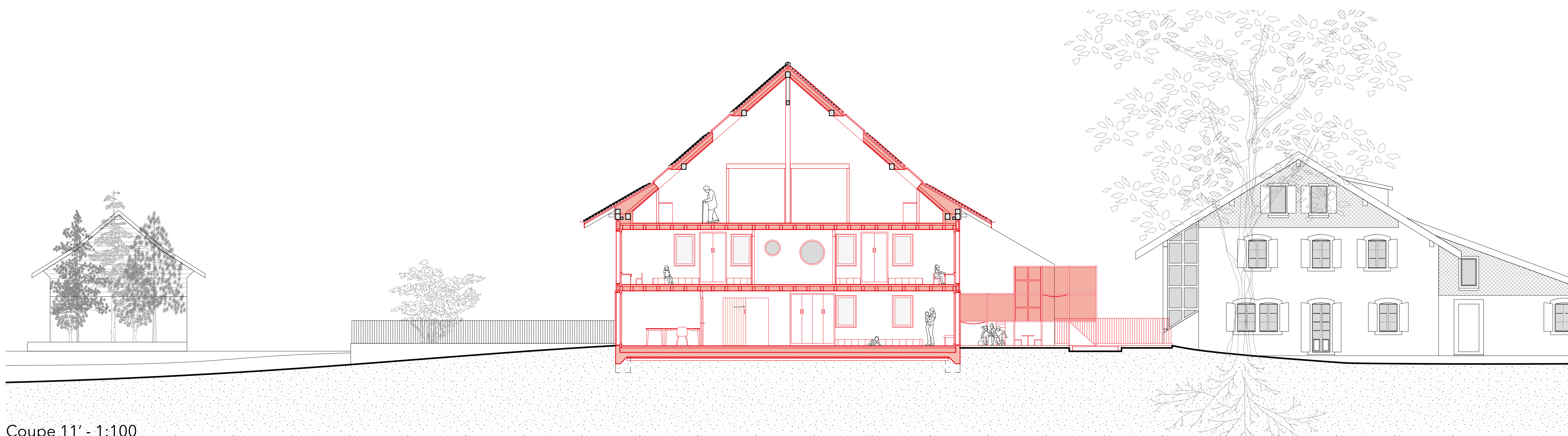
Coupe 11' - 1:100
