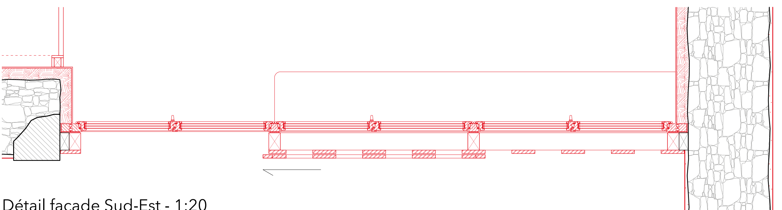
Détail façade Sud-Est - 1:20
