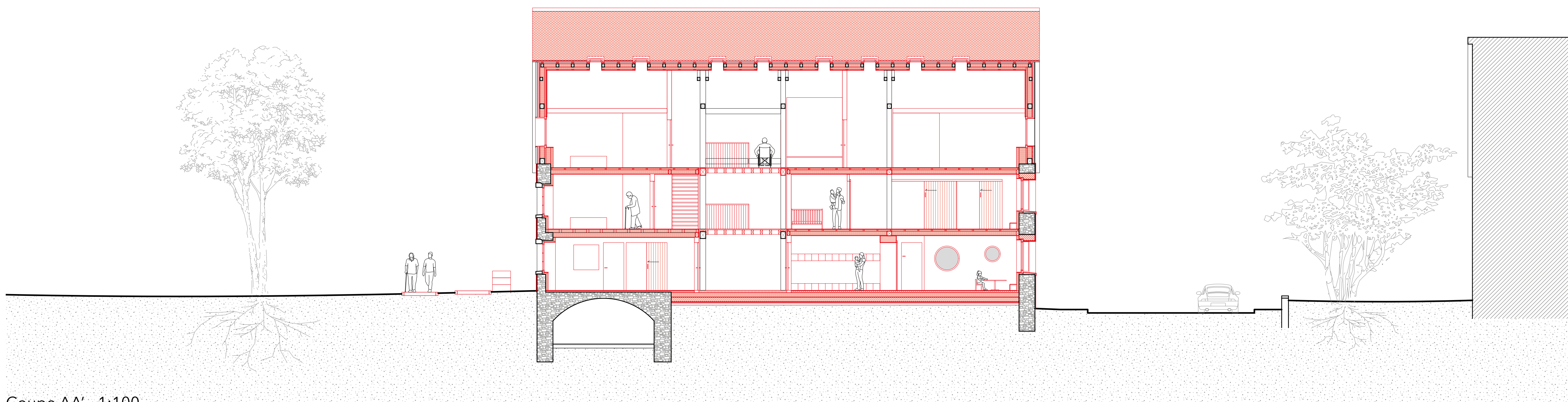
Coupe AA' - 1:100
