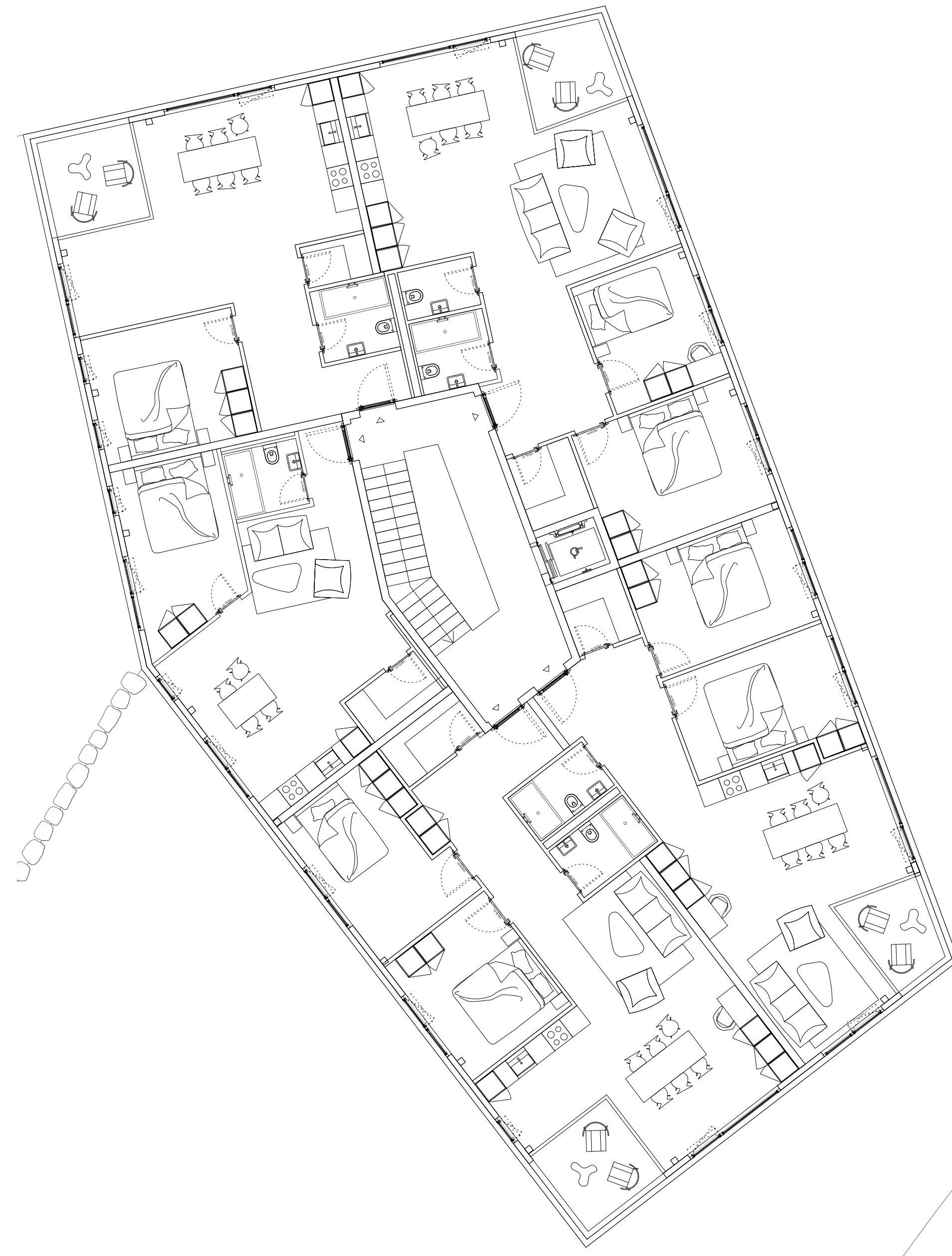
plan étages +5, +6, +7, echelle 1:100
