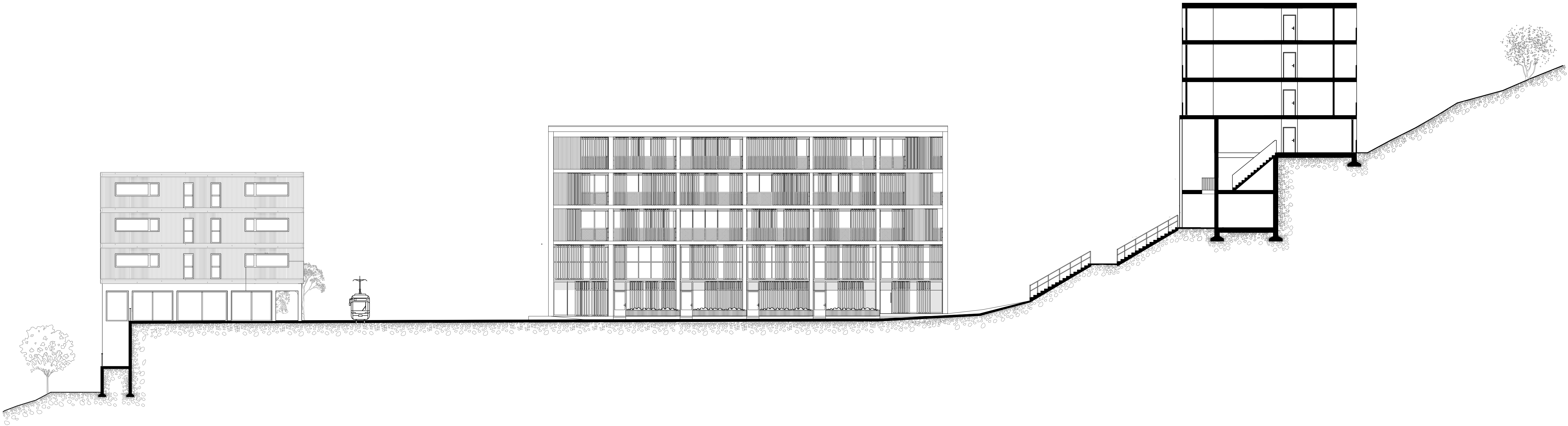
Coupe transversale Ouest 1:200
