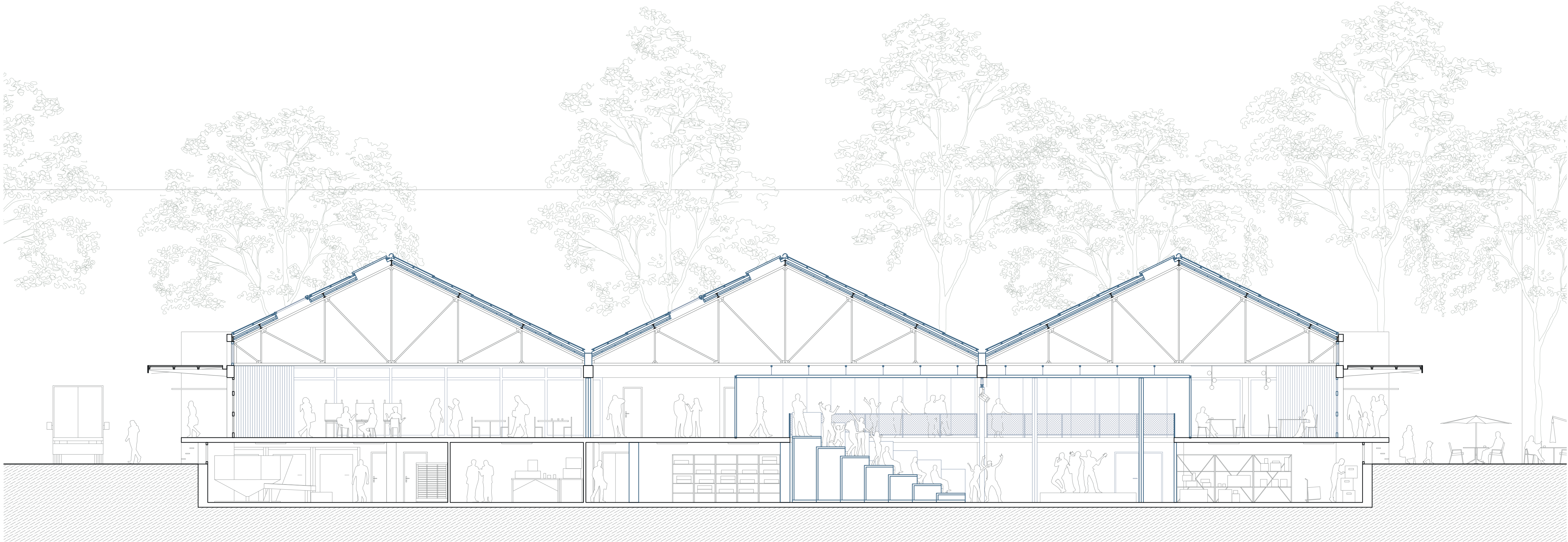
Coupe longitudinale 1:100
