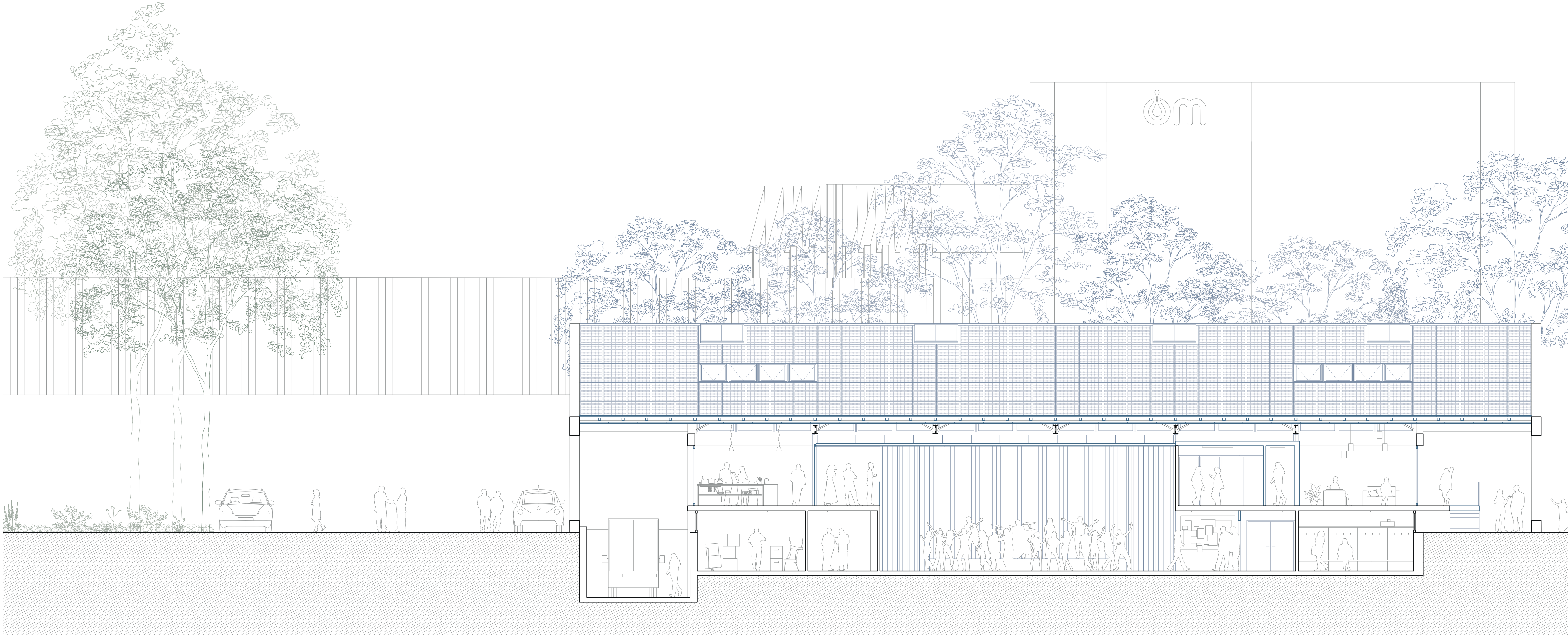
Coupe transversale BB' 1:100
