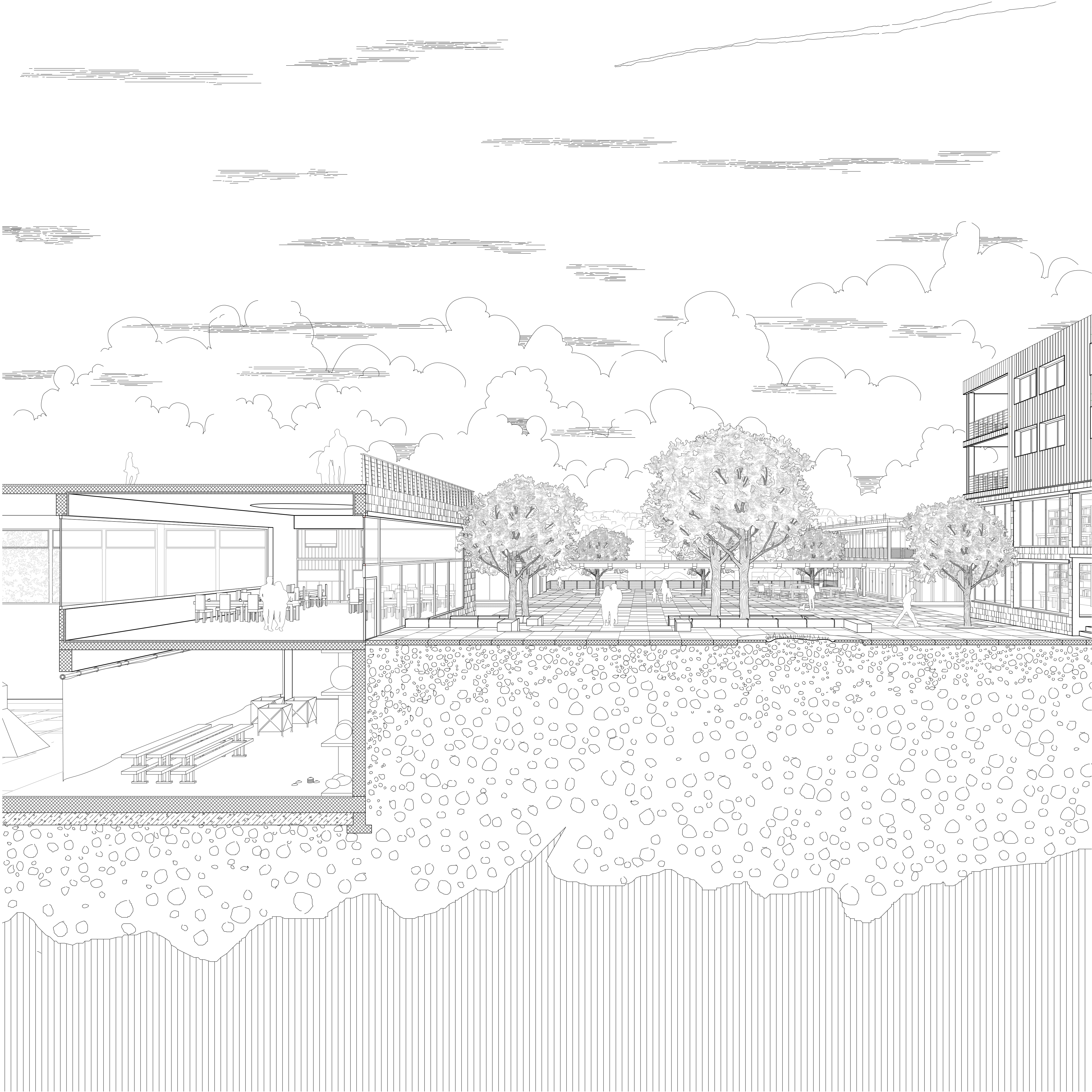
Coupe perspective
