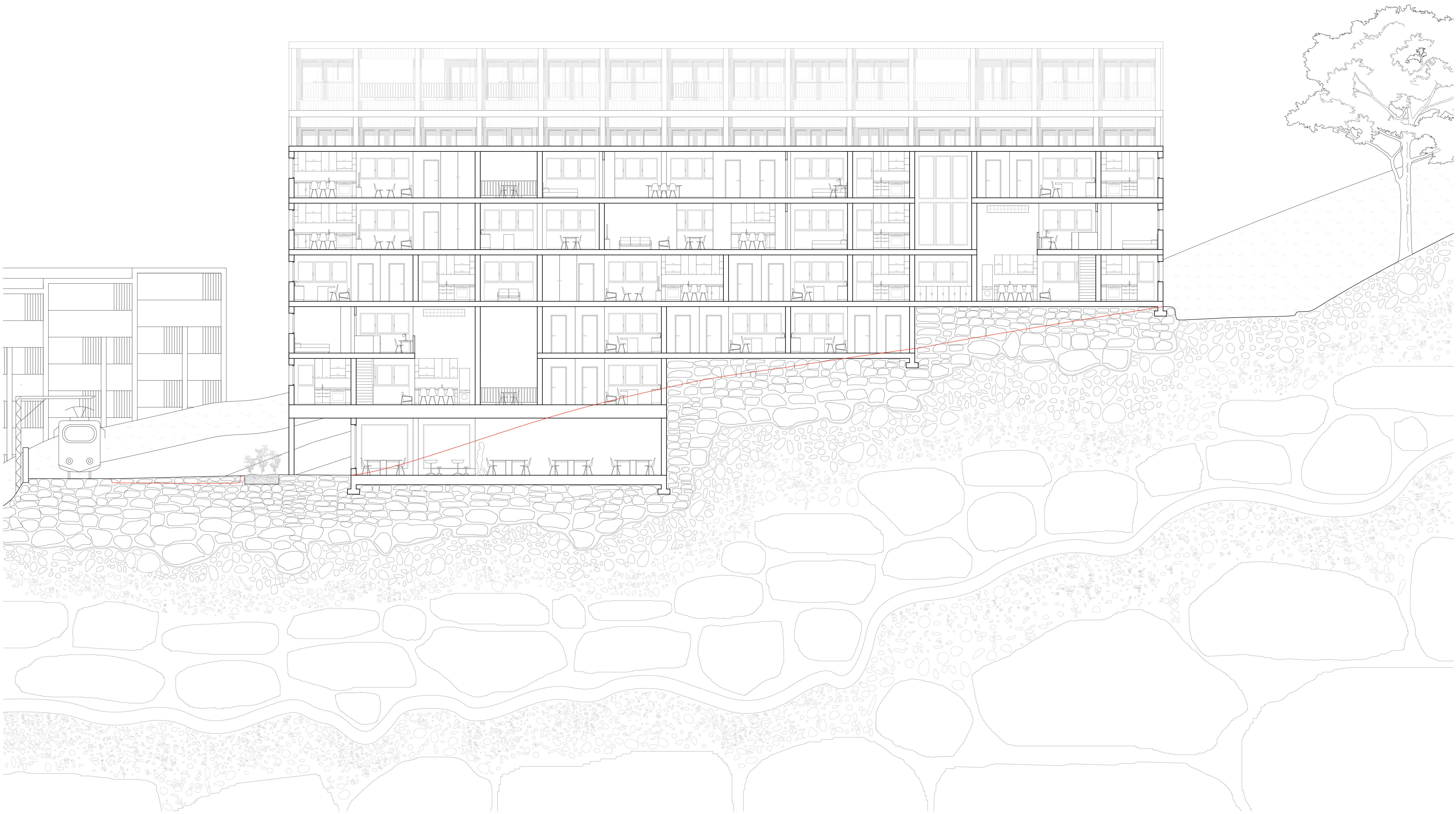
Coupe transversale ouest 1:200
