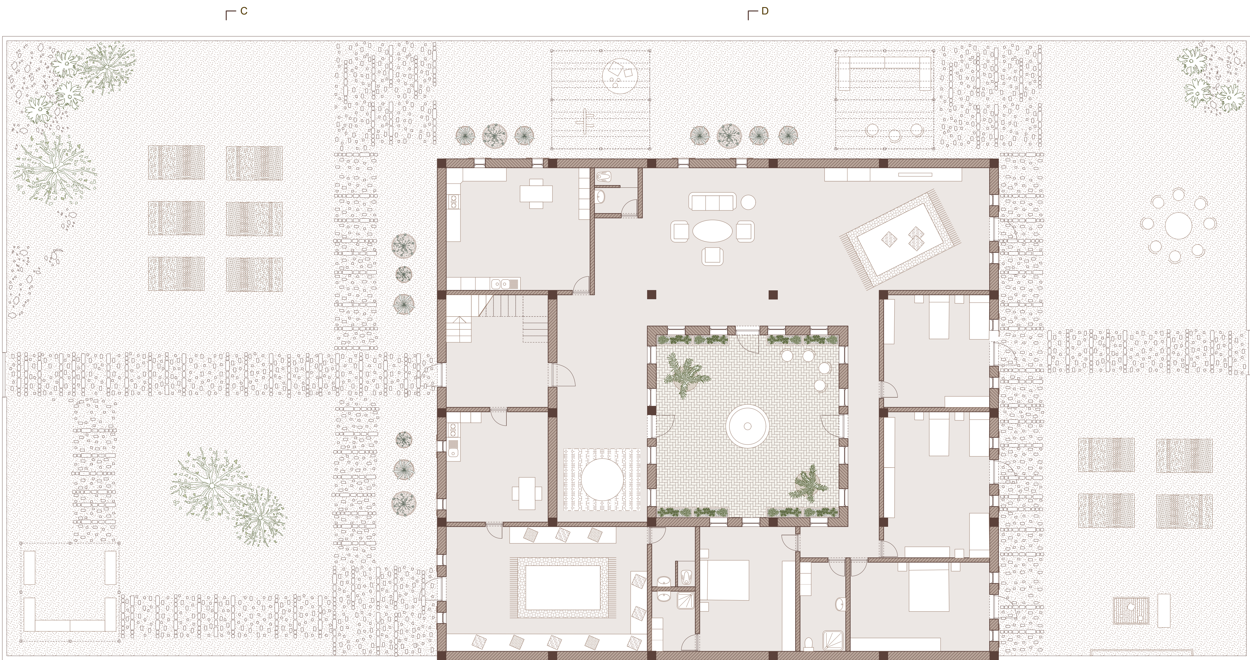
plan rez-de-chaussée
