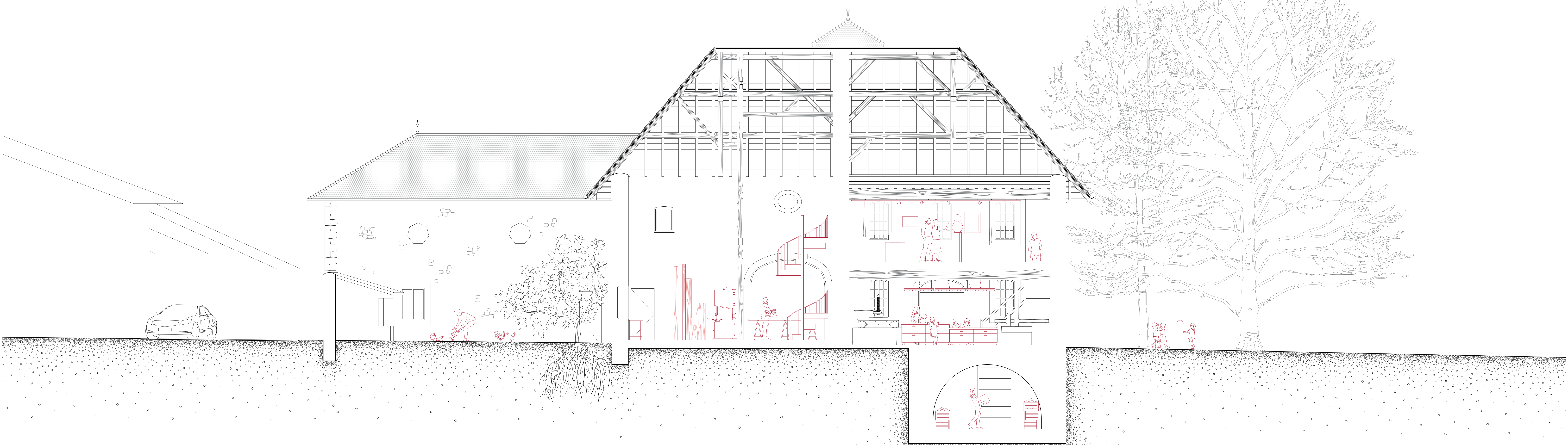
Coupe A-A' 1:50
