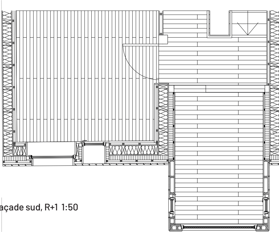
élévation façade sud 1:50
