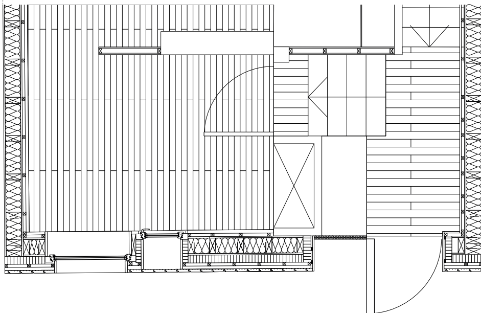
plan détail façade sud, R+0 1:50
