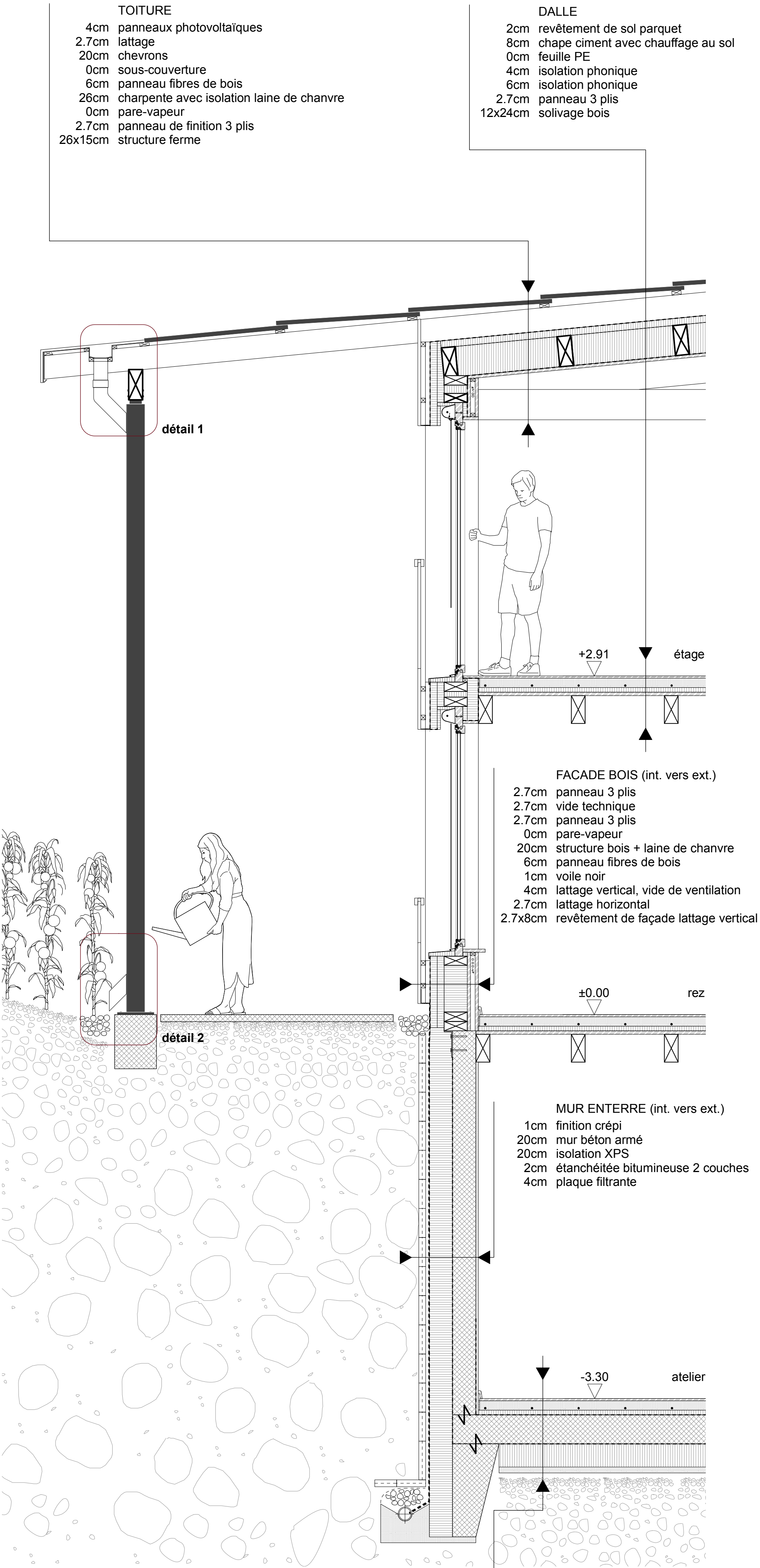
Travée, échelle 1:25
