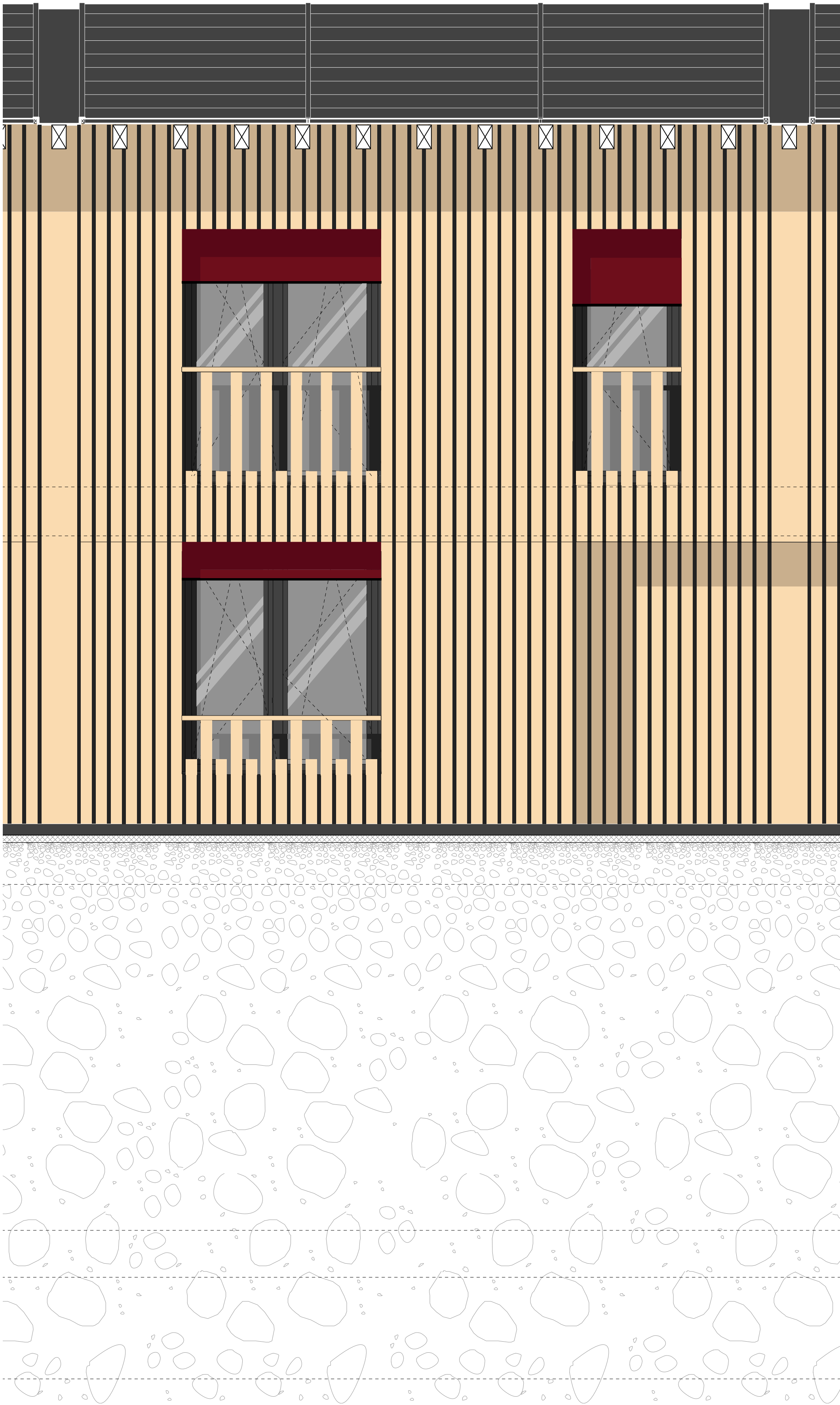
Elévation, échelle 1:25
