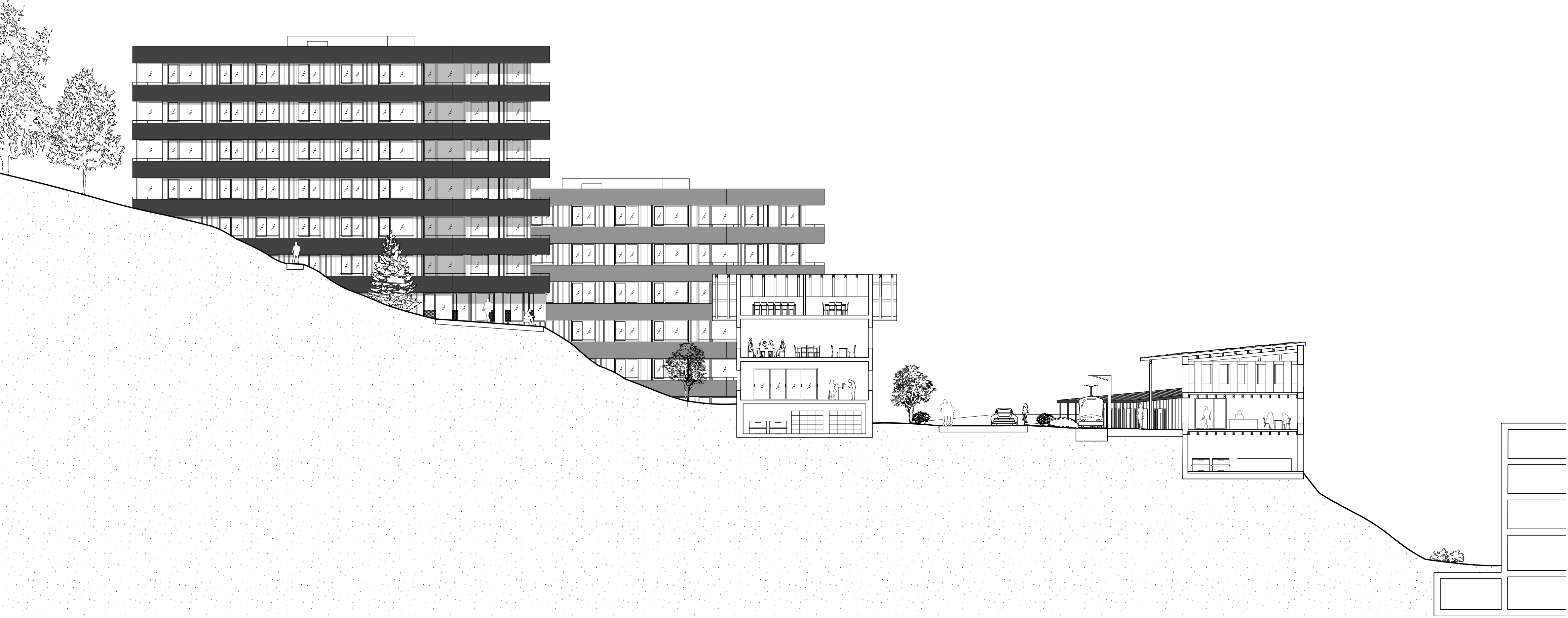
Coupe longitudinale 1:500
