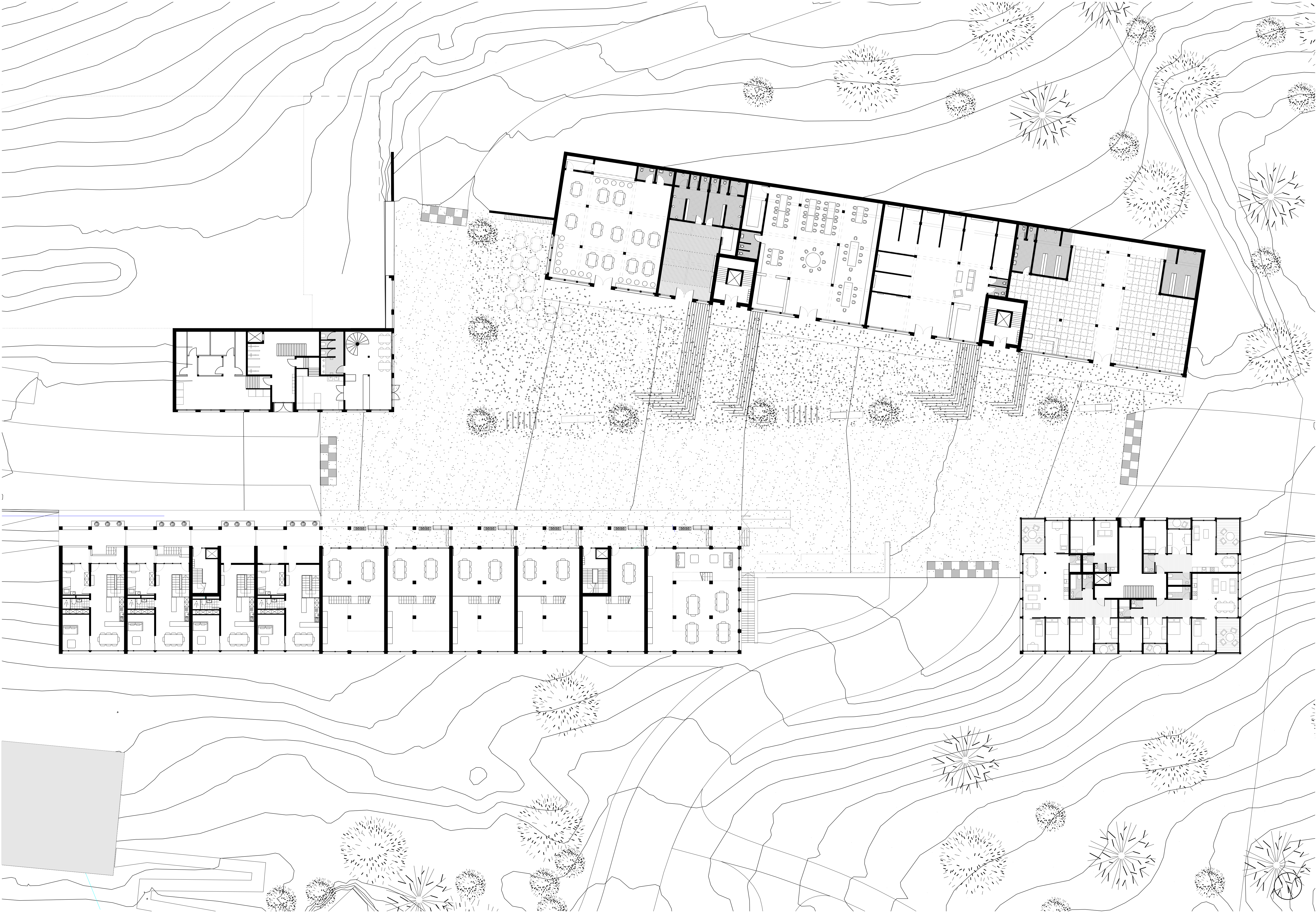
Plan des rez-de-chaussée 1:200
