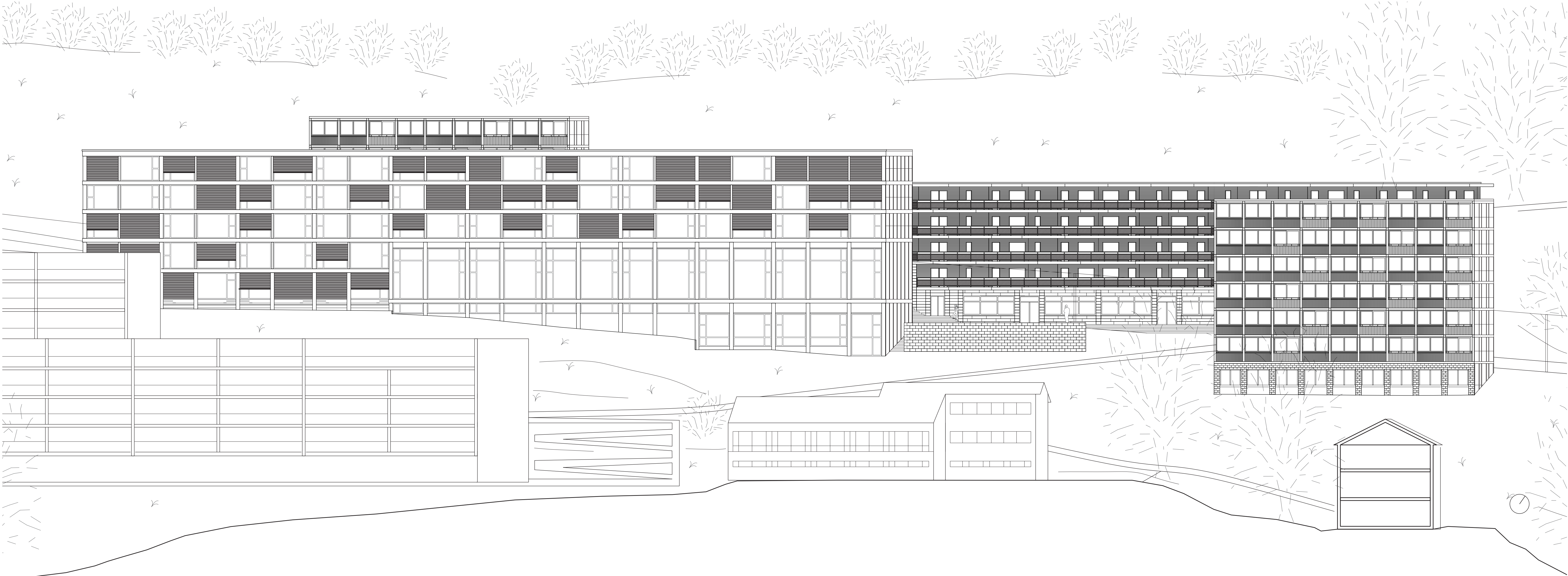
coupe longitudinale 1:200
