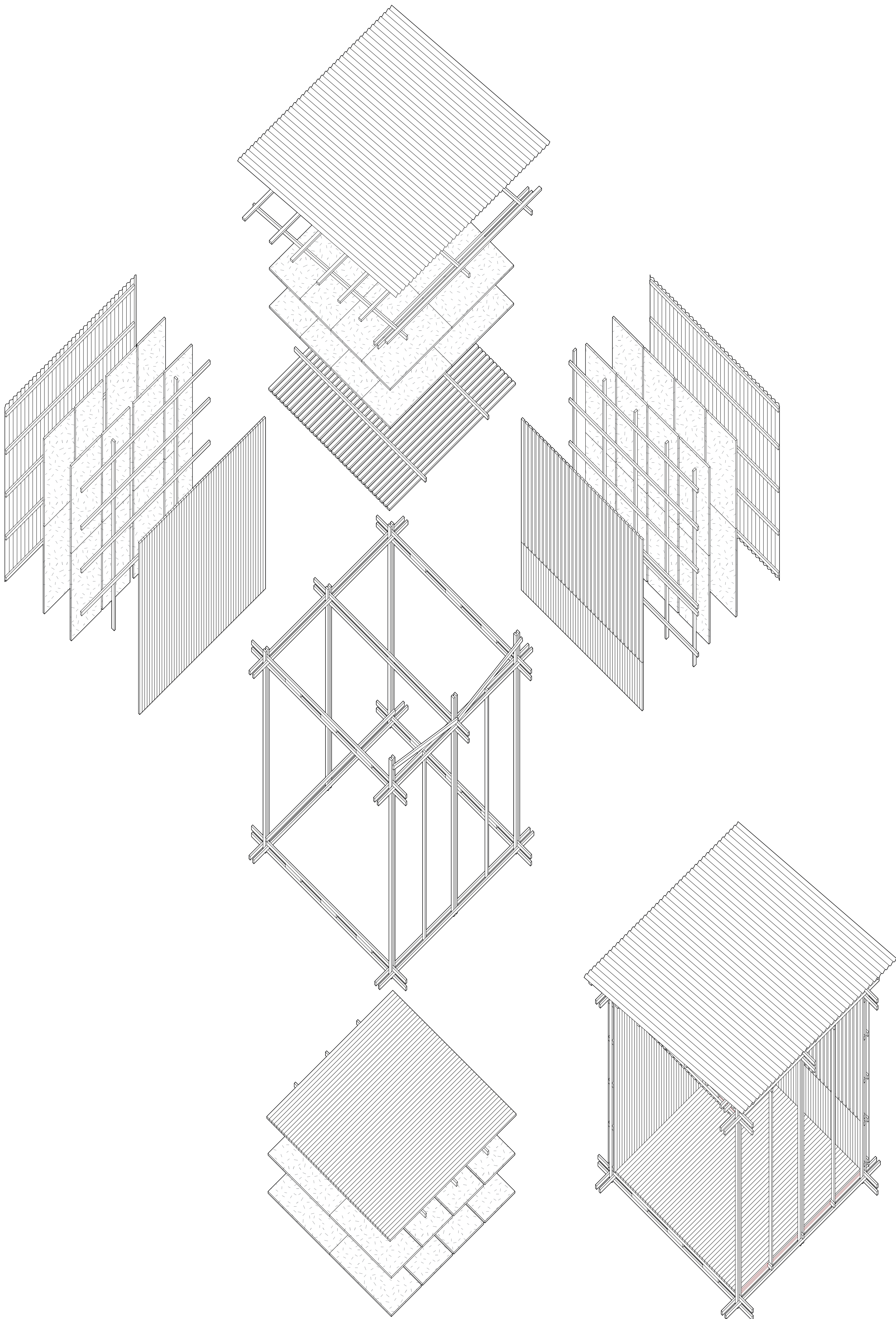
Montage des planchers, plafonds, parois, isolation et revêtements - 1:33
