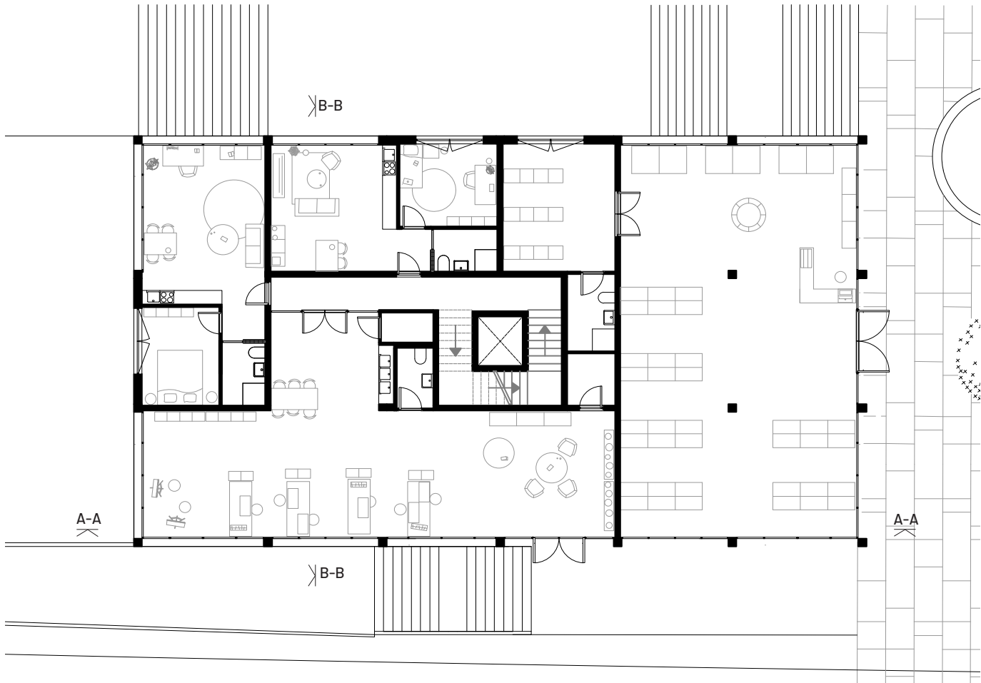
Plan rez-de-chaussée 1:200
