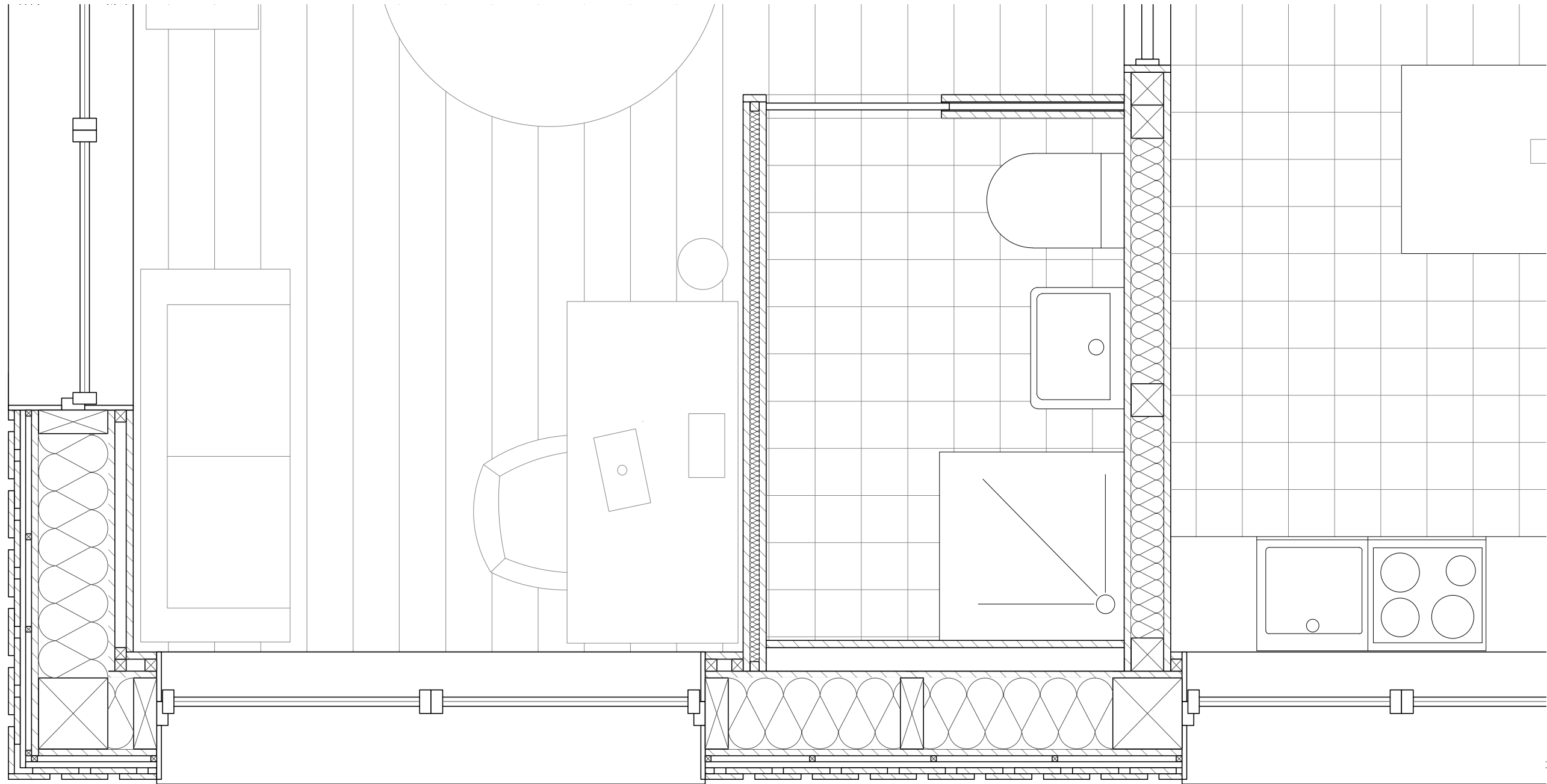
Plan détail 1:20
