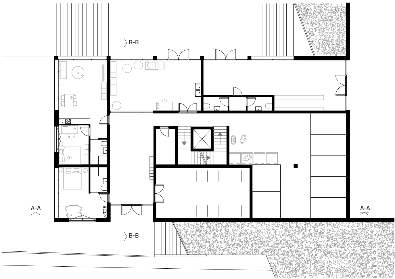
Plan sous-sol 1:200
