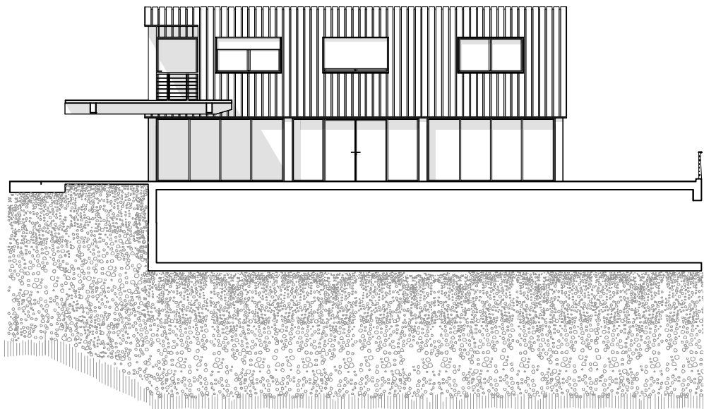
Élévation est 1:200
