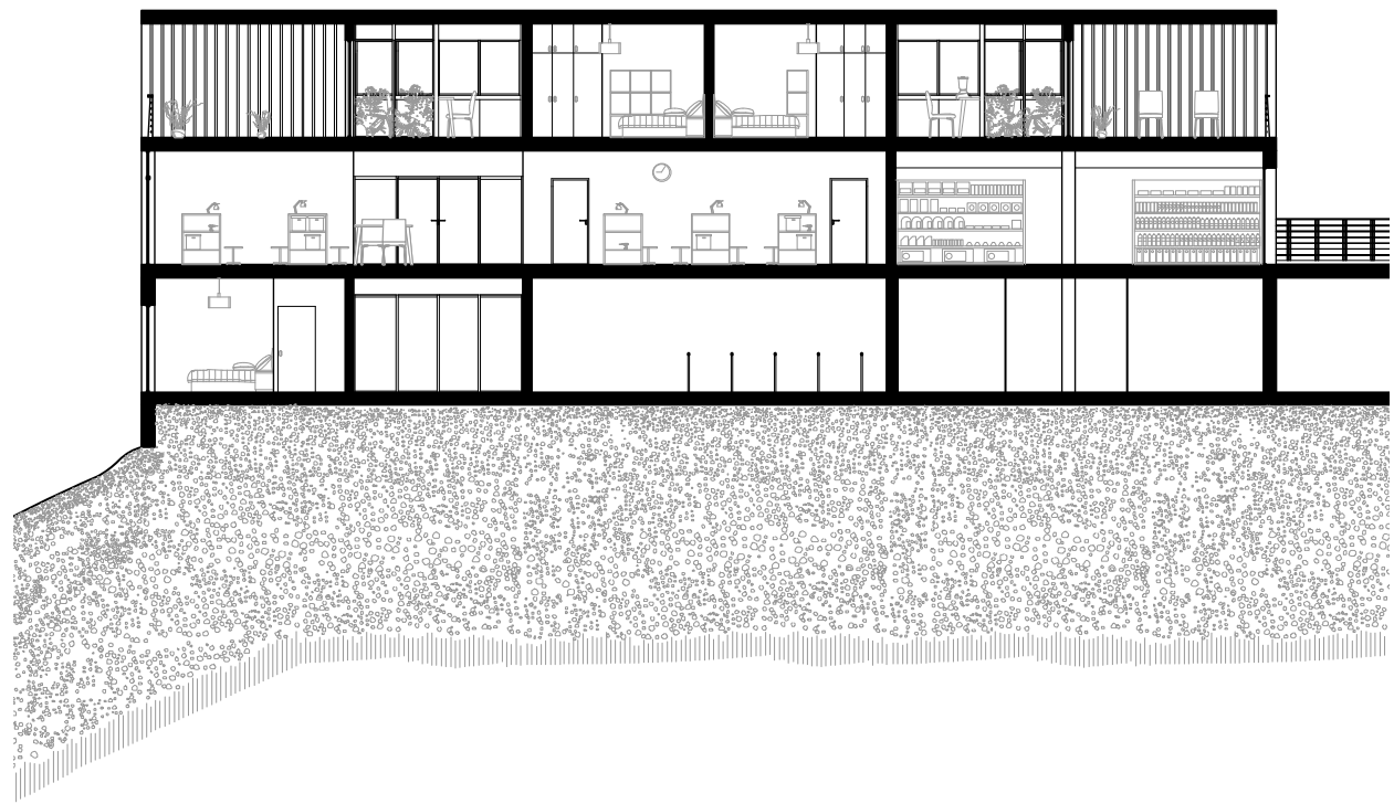
Coupe A-A 1:200
