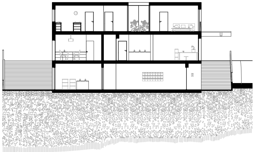
Coupe B-B 1:200
