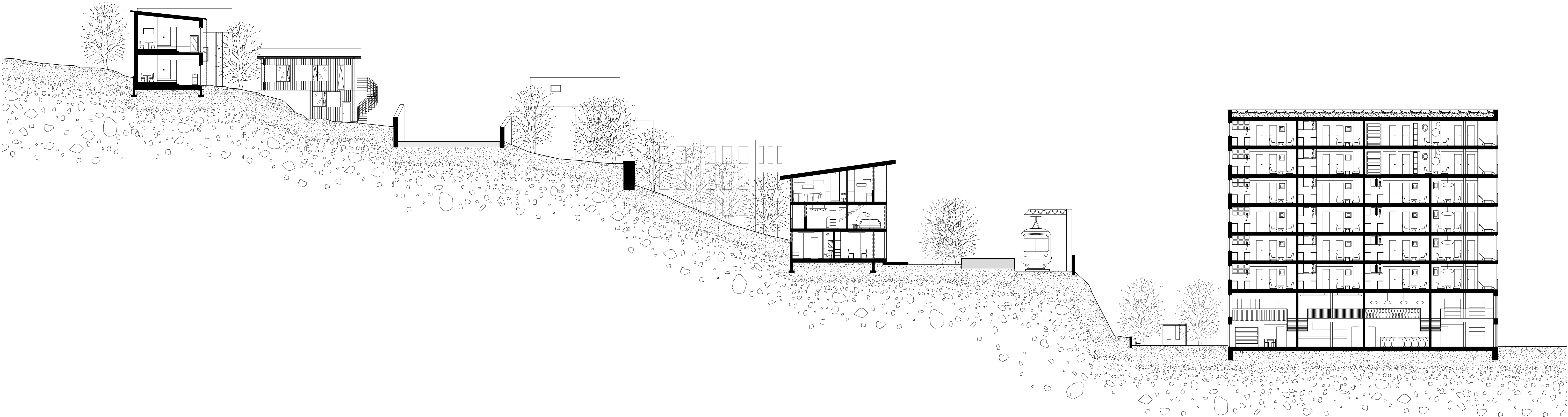
Coupe transversal 1:200
