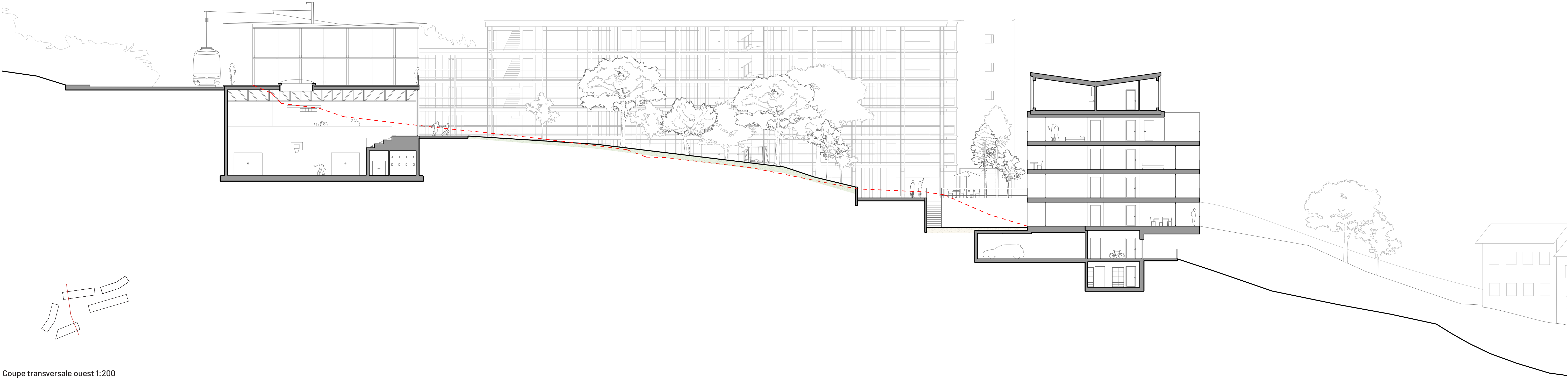
Coupe transversale ouest 1:200
