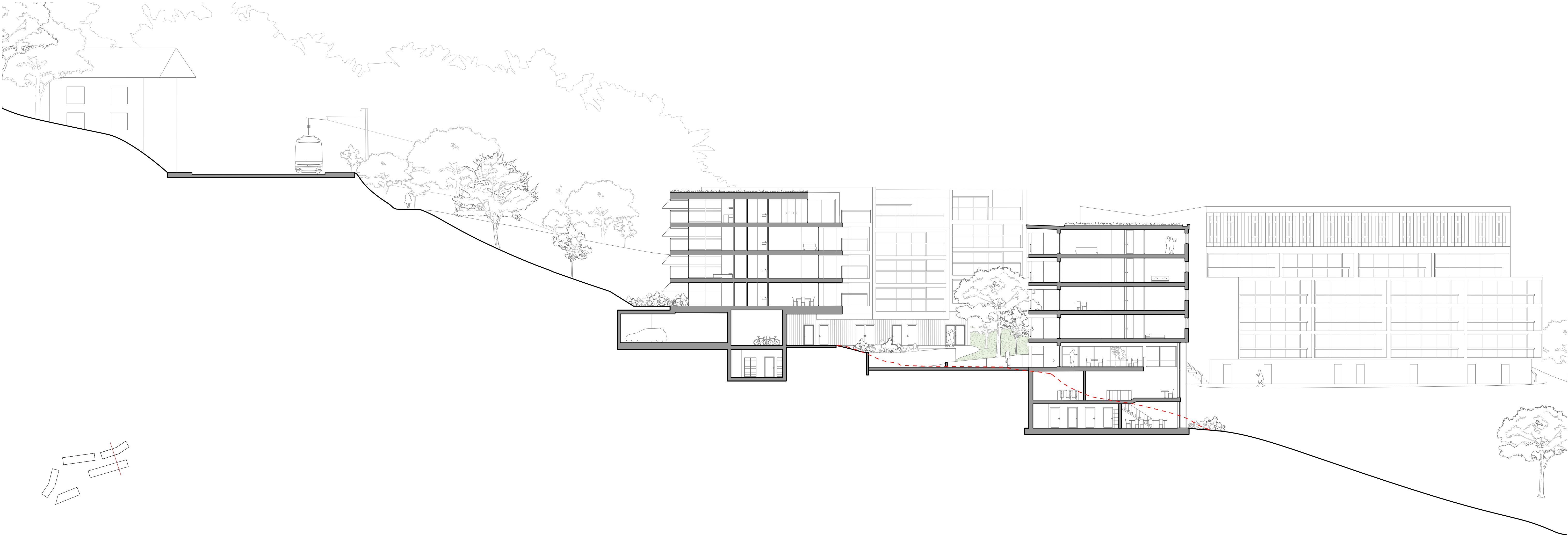
Coupe transversale ouest 1:200
