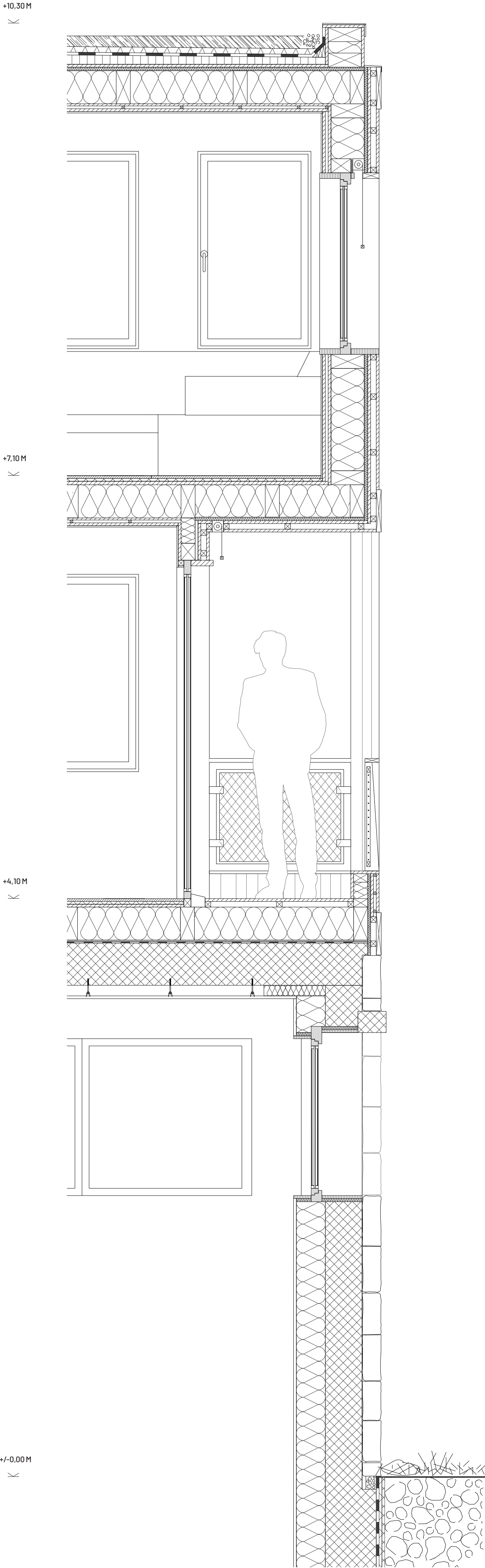
Coupe détail 1:20
